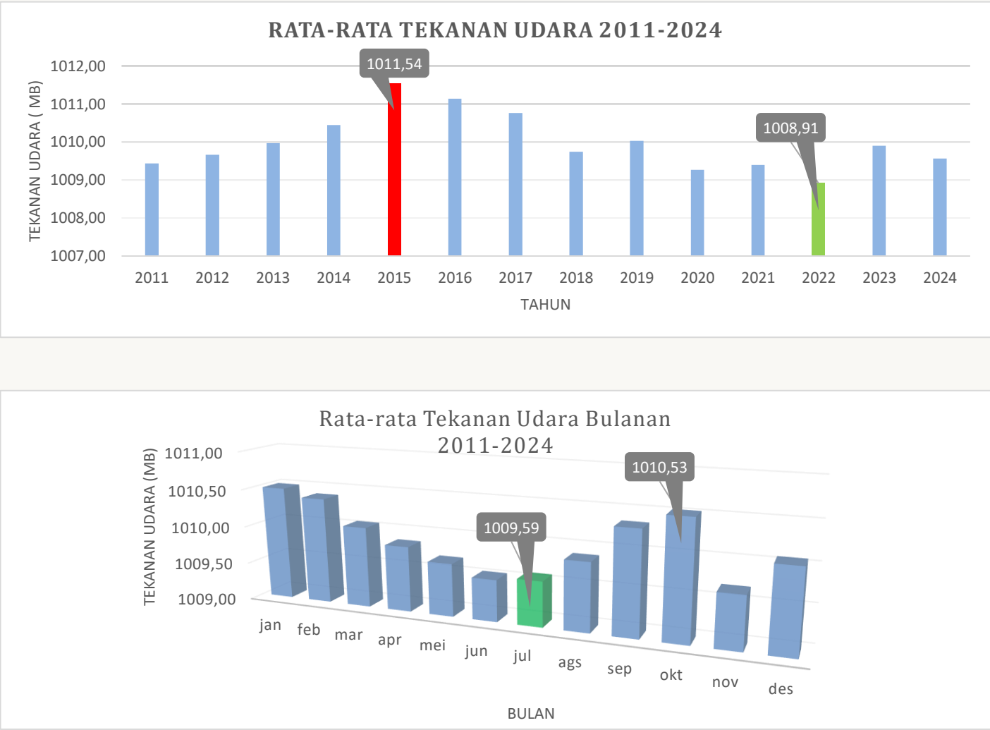
Gambar 3.1.5 Grafik Rata-Rata Tekanan Udara
