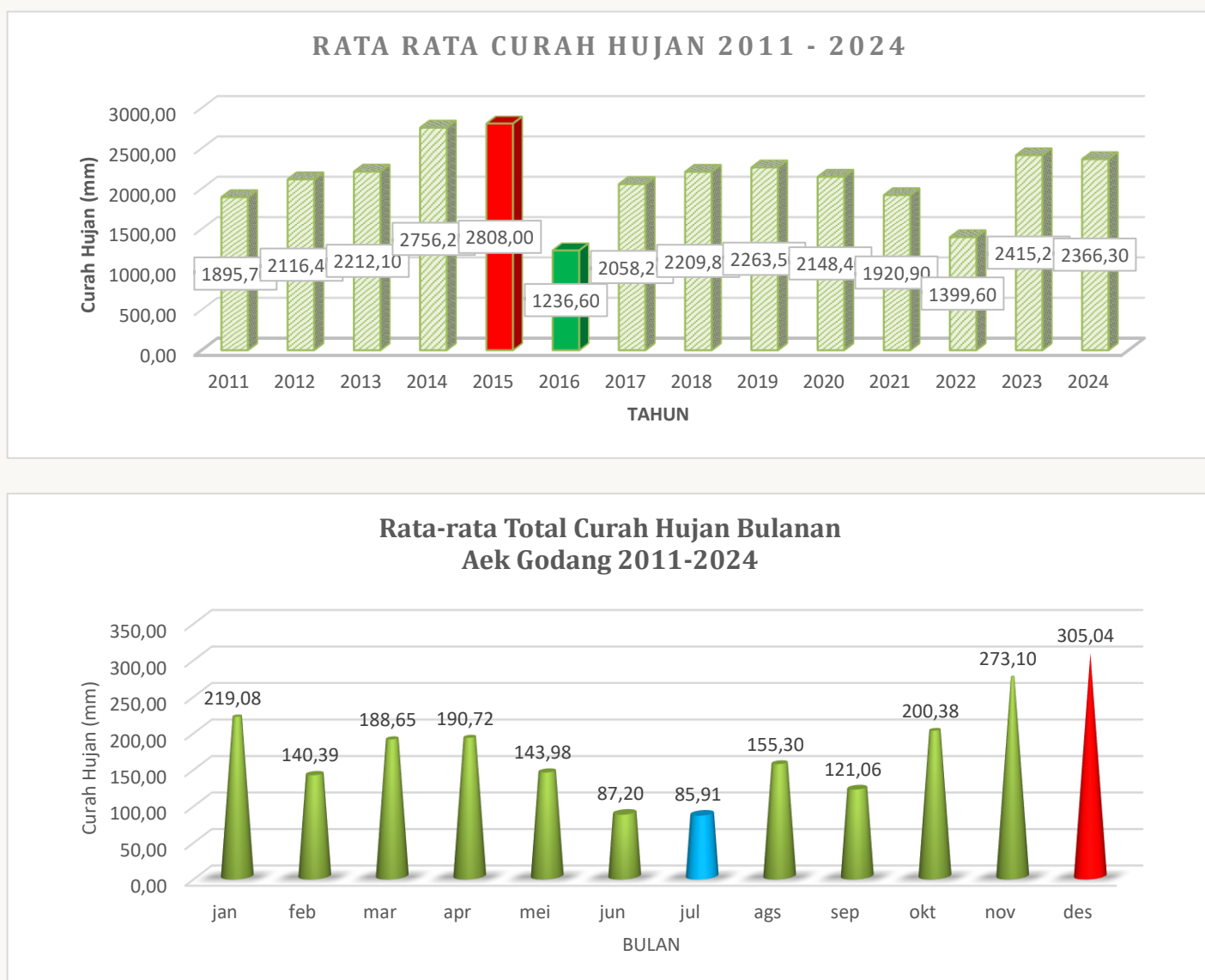
Gambar 3.1.3 Grafik Rata-Rata Curah Hujan
