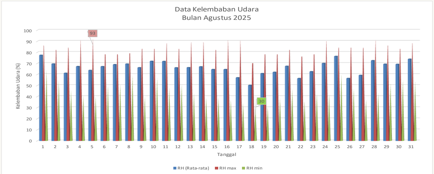
Gambar 2.1.5 Grafik Kelembaban Udara Bulan Agustus 2025
