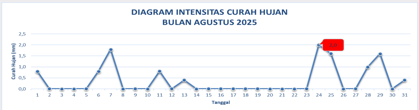
Gambar 2.1.3. Intensitas Curah Hujan Bulan Agustus 2025
