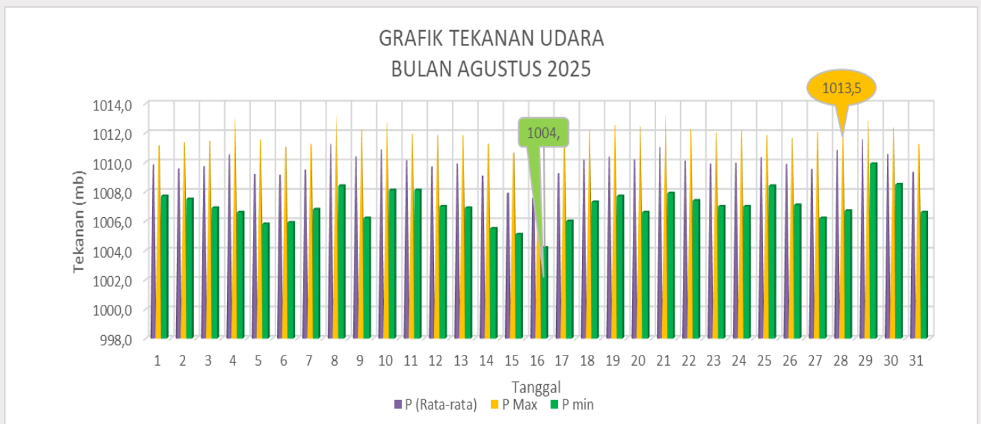
Gambar 2.1.4. Tekanan Udara Bulan Agustus 2025
