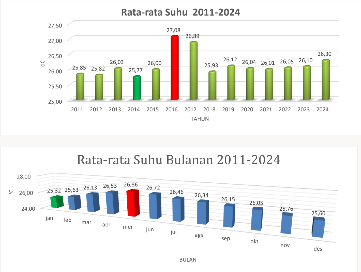
Gambar 3.1.2 Grafik Rata-Rata Suhu Udara
