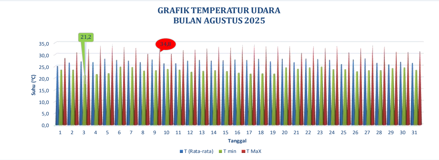
Gambar 2.1.1 Grafik Suhu Udara Bulan Agustus 2025
