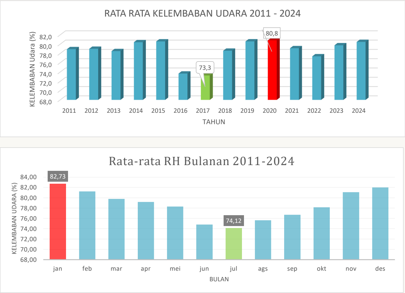
Gambar 3.1.4 Grafik Rata-Rata Kelembaban Udara
