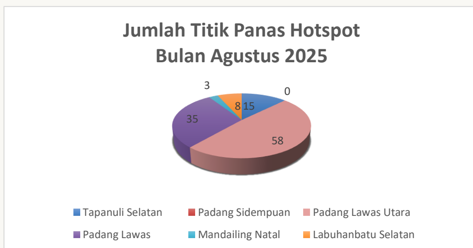
Gambar 2.1.7. Grafik Titik Panas Hotspot Bulan Agustus 2025
