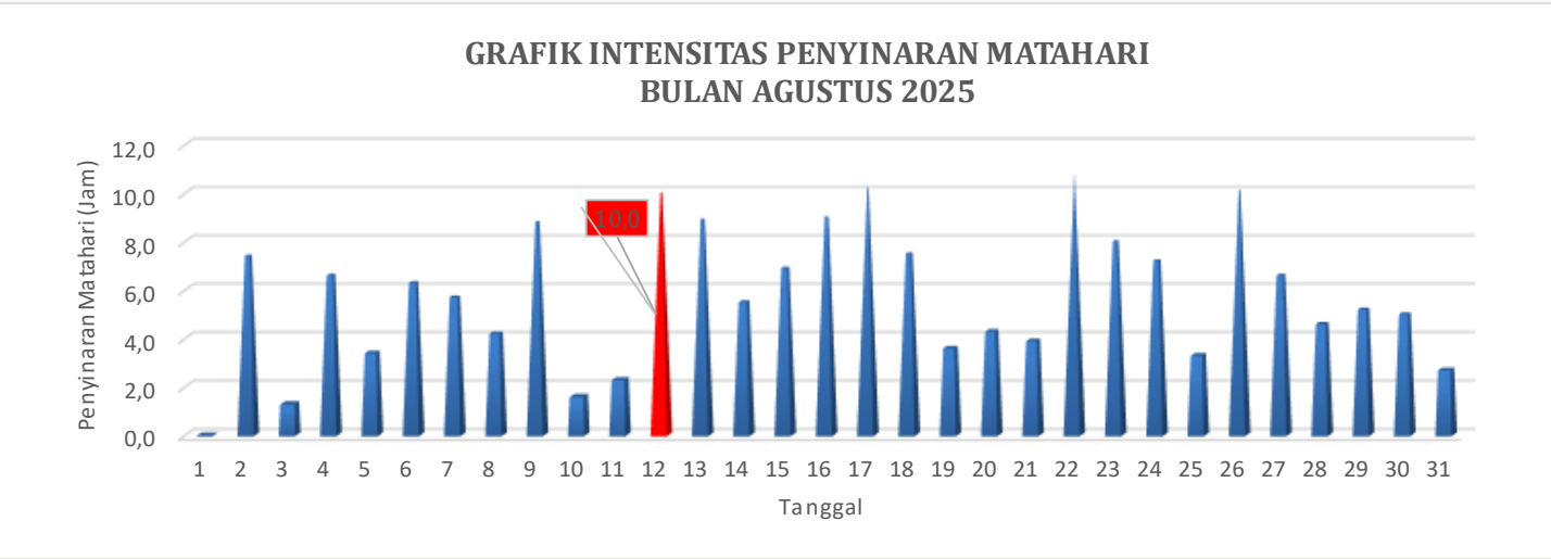
Gambar 2.1.2. Grafik Durasi Penyinaran Matahari Bulan Agustus 2025
