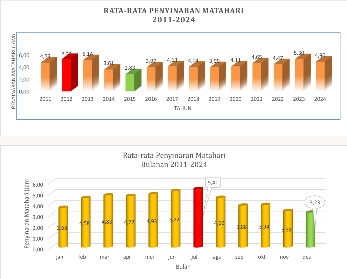
Gambar 3.1.1 Grafik Rata-Rata Penyinaran Matahari
