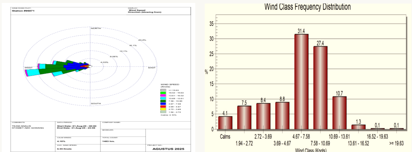
Gambar 2.1.6. Grafik Arah dan Kecepatan Angin Bulan Agustus 2025
