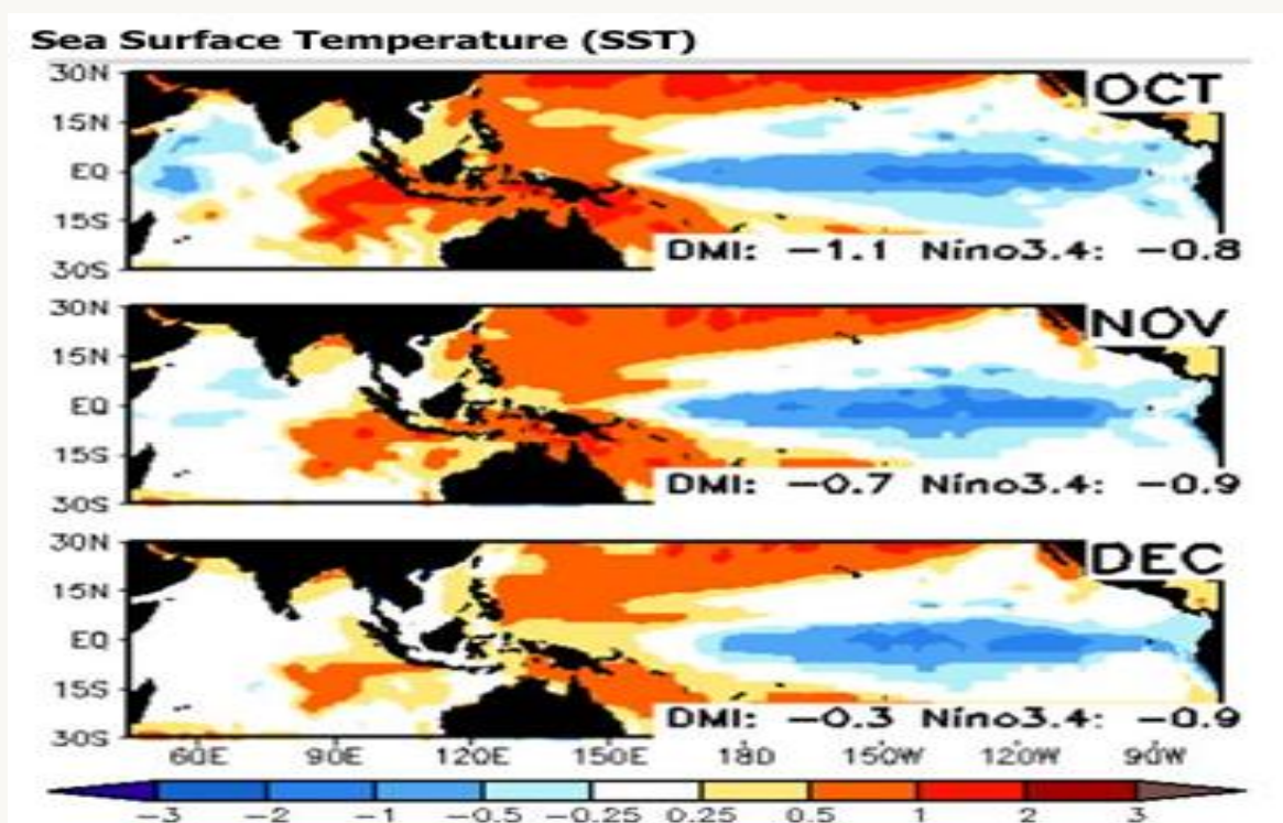
Gambar 2.1.1.A Prediksi Anomali SST
