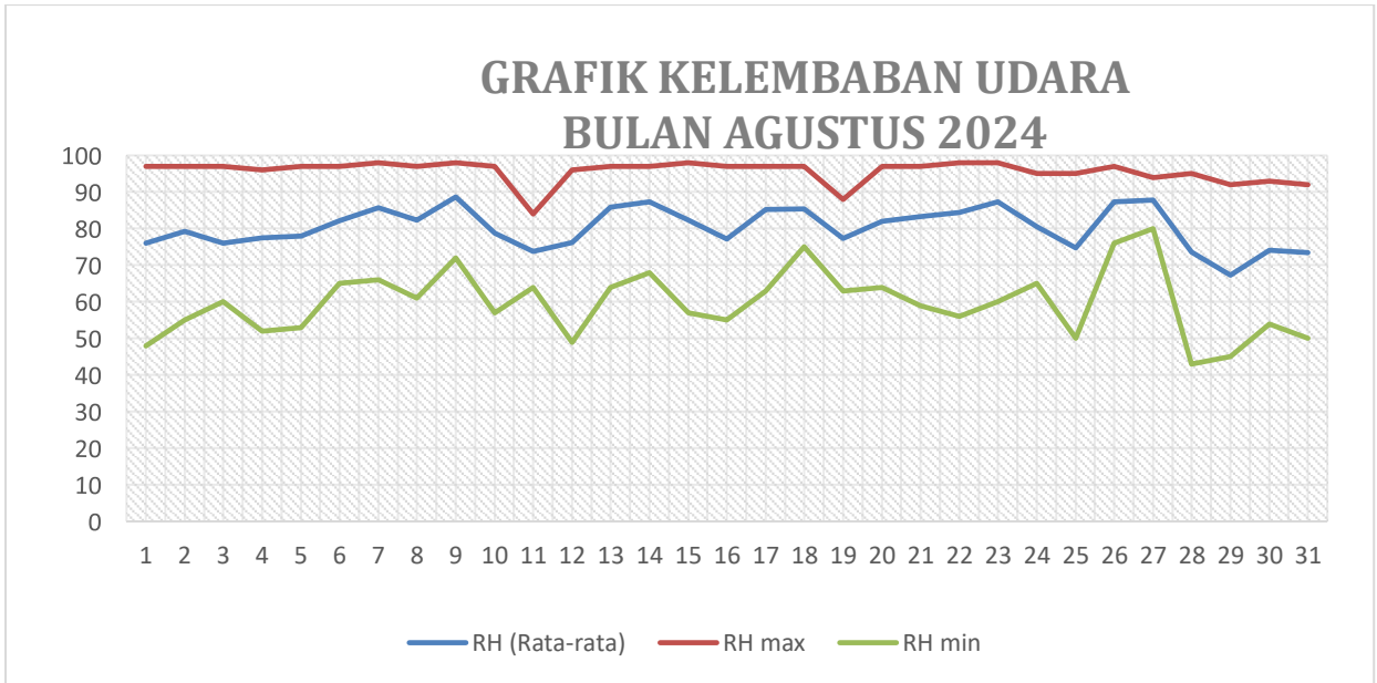
Gambar 2.1.5.1 Grafik Kelembaban Udara Bulan Agustus 2024
