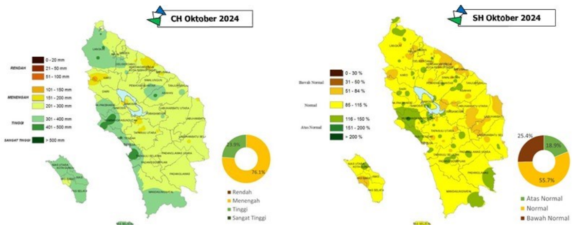
Gambar 2.5.1 Prakiraan Curah Hujan dan Sifat Hujan Oktober 2024
