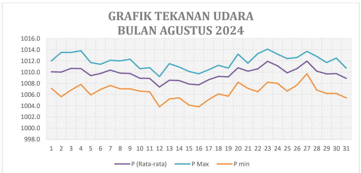
Gambar 2.1.4.1 Grafik Tekanan Udara Bulan Agustus 2024
