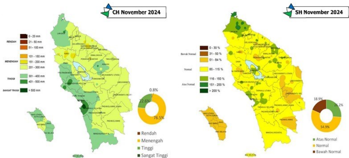
Gambar 2.5.2 Prakiraan Curah Hujan dan Sifat Hujan November 2024
