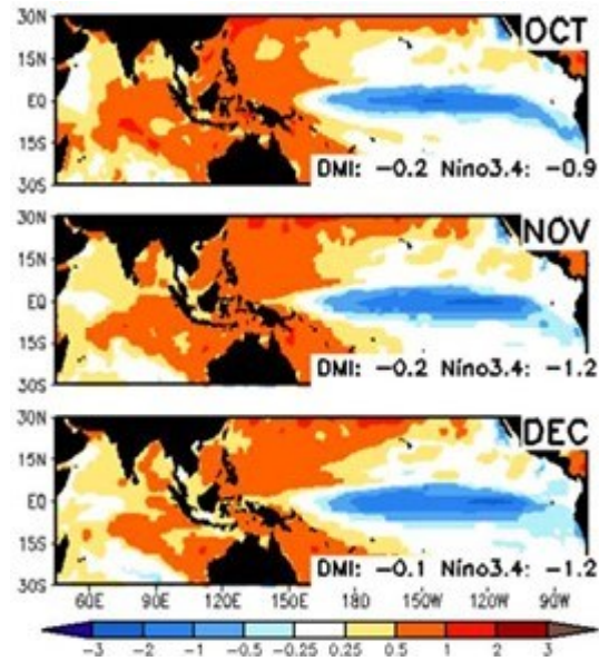
Gambar. 2.2.1 Prediksi Anomali SST
