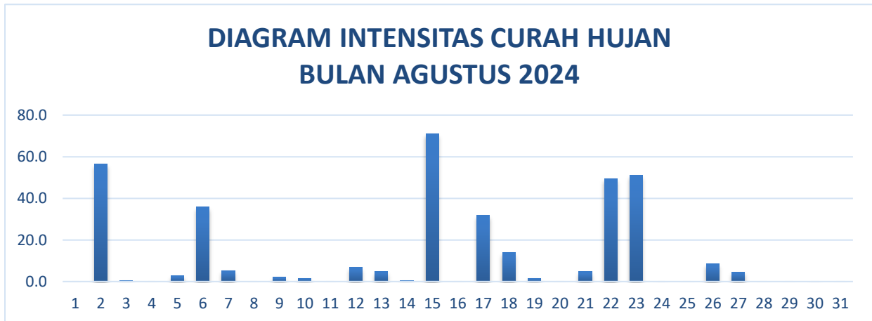
Gambar 2.1.3.2 Intensitas Curah Hujan Bulan Agustus 2024
