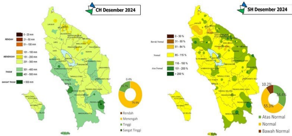
Gambar 2.5.3 Prakiraan Curah Hujan dan Sifat Hujan Desember 2024
