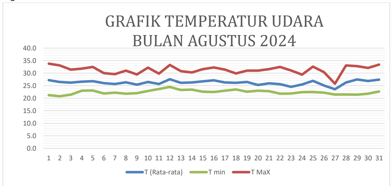
Gambar 2.1.1.1 Grafik Suhu Udara Bulan Agustus 2024
