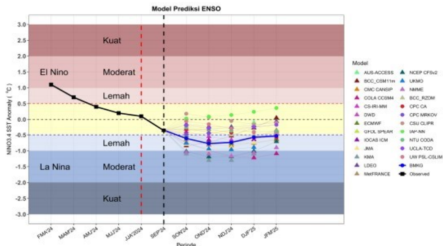
Gambar. 2.2.2 Prediksi ENSO
