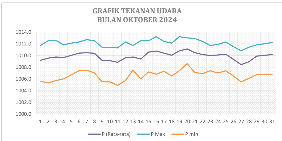
Gambar 2.1.4.1 Grafik Tekanan Udara Bulan Oktober 2024
