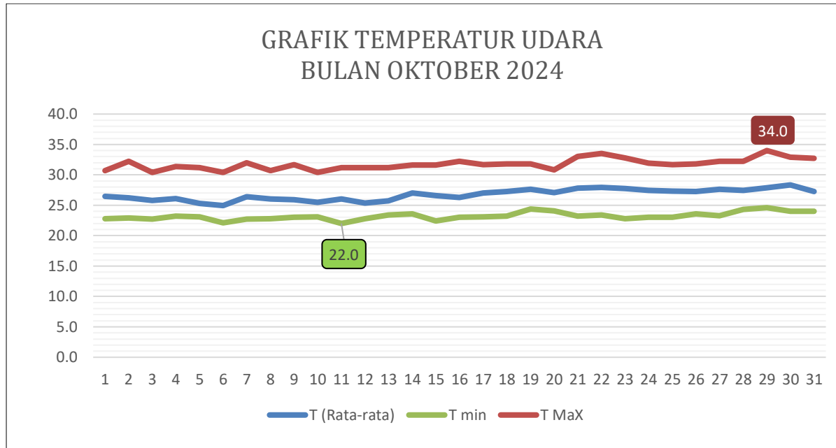
Gambar 2.1.1.1 Grafik Suhu Udara Bulan Oktober 2024
