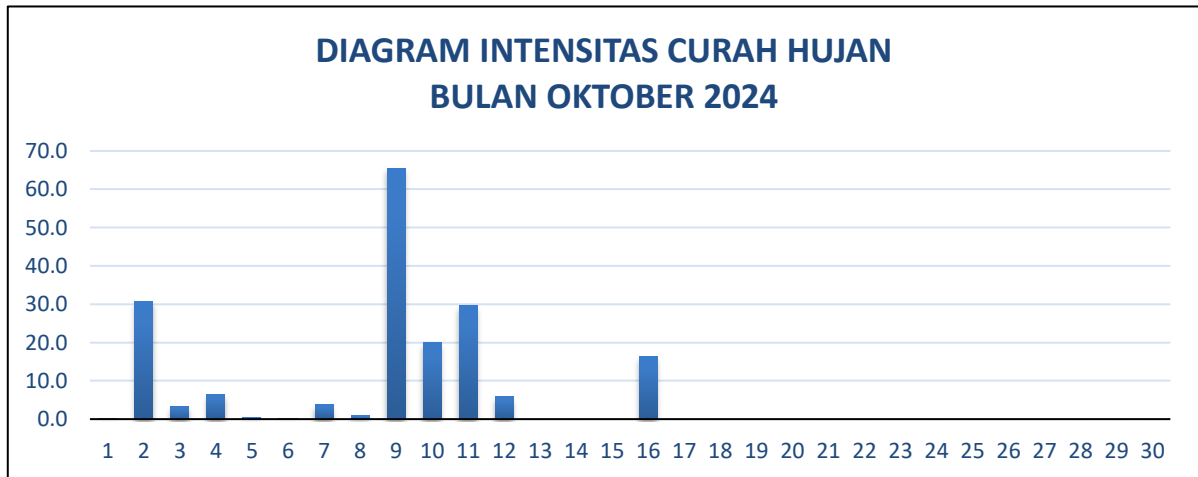
Gambar 2.1.3.2 Intensitas Curah Hujan Bulan Oktober 2024
