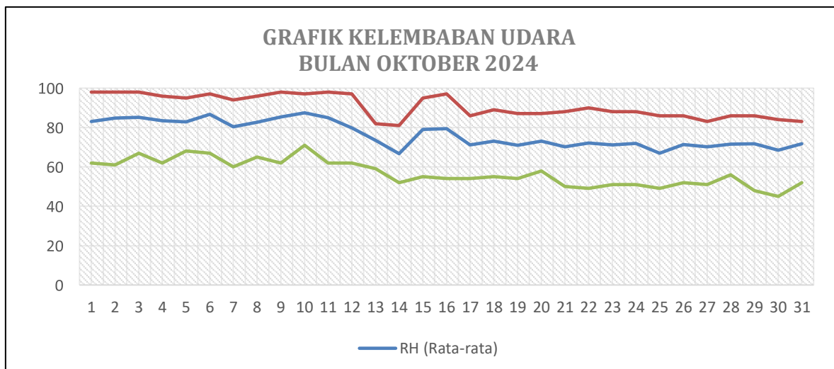
Gambar 2.1.5.1 Grafik Kelembaban Udara Bulan Oktober 2024
