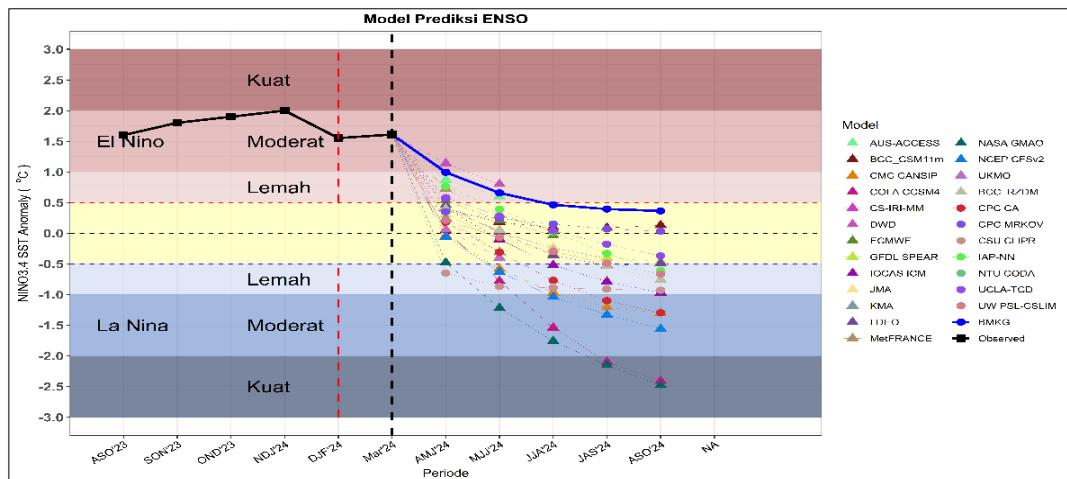
Gambar. 2.2.2 Prediksi ENSO
