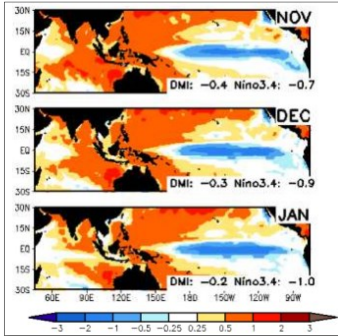
Gambar. 2.2.1 Prediksi Anomali SST
