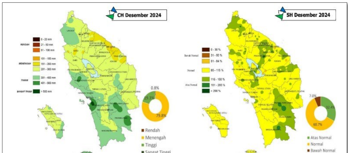
Gambar 2.5.2 Prakiraan Curah Hujan dan Sifat Hujan Desember 2024
