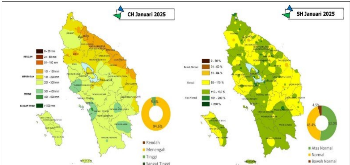
Gambar 2.5.3 Prakiraan Curah Hujan dan Sifat Hujan Januari 2025
