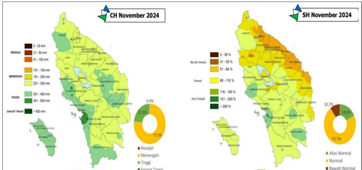
Gambar 2.5.1 Prakiraan Curah Hujan dan Sifat Hujan November 2024
