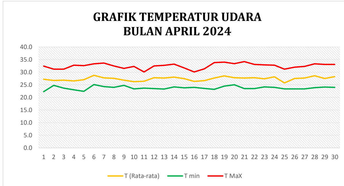
Gambar 2.1.1.1 Grafik Suhu Udara Bulan April 2024
