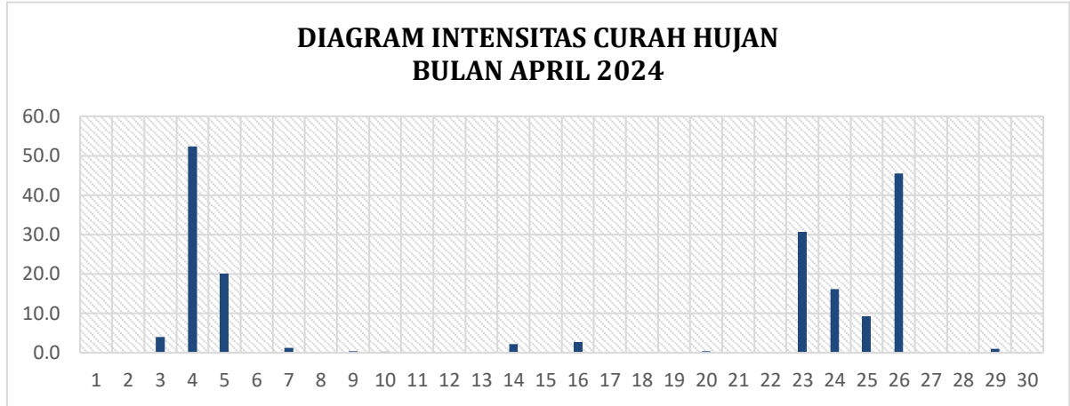
Gambar 2.1.3.2 Intensitas Curah Hujan Bulan April 2024
