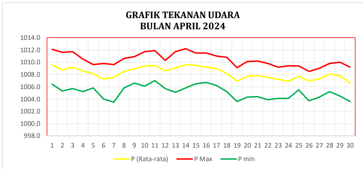
Gambar 2.1.4.1 Grafik Tekanan Udara Bulan April 2024
