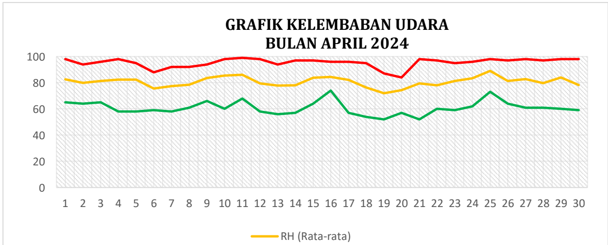
Gambar 2.1.5.1 Grafik Kelembaban Udara Bulan April 2024
