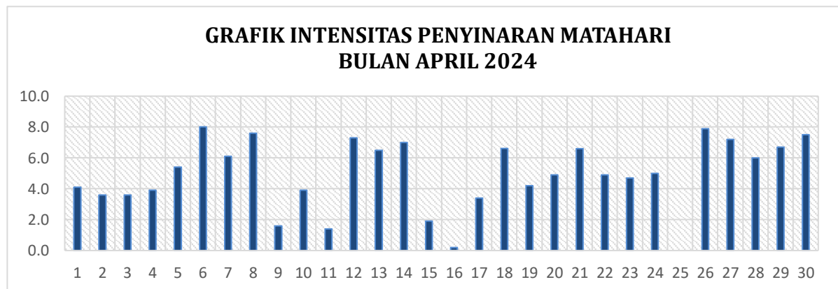
Gambar 2.1.2.1 Grafik Durasi Penyinaran Matahari Bulan April 2024
