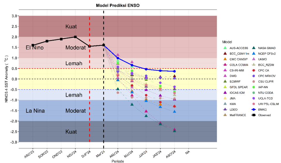
Gambar. 2.2.2 Prediksi ENSO
