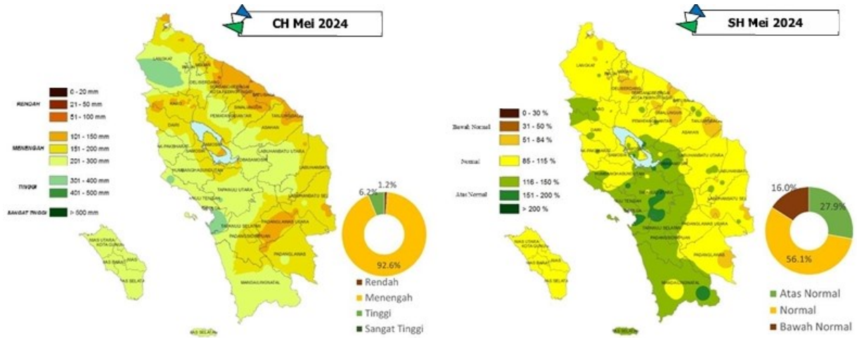
Gambar 2.5.1 Prakiraan Curah Hujan dan Sifat Hujan Mei 2024
