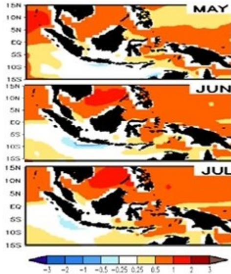
Gambar. 2.2.1 Prediksi Anomali SST
