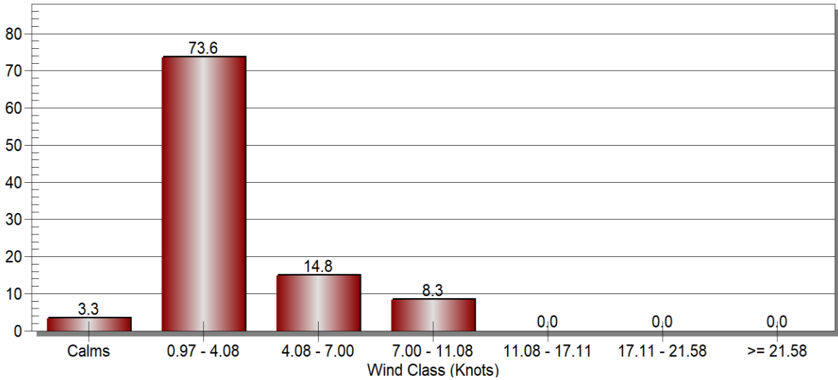
Gambar 2.1.6.1 Diagram Arah dan Kecepatan Angin Bulan April 2024
