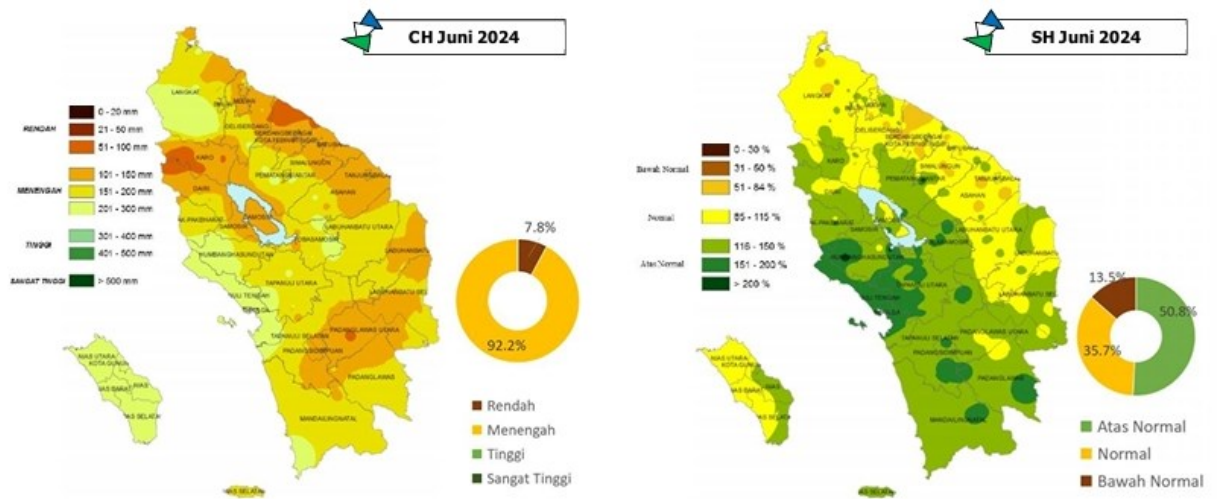
Gambar 2.5.2 Prakiraan Curah Hujan dan Sifat Hujan Juni 2024
