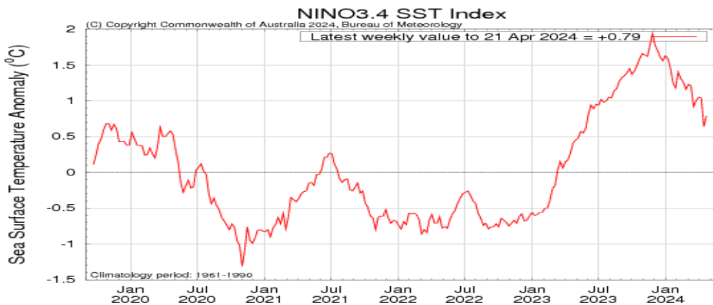
Gambar. 1.2.1 Indeks NINO 3.4 Bulan April 2024
