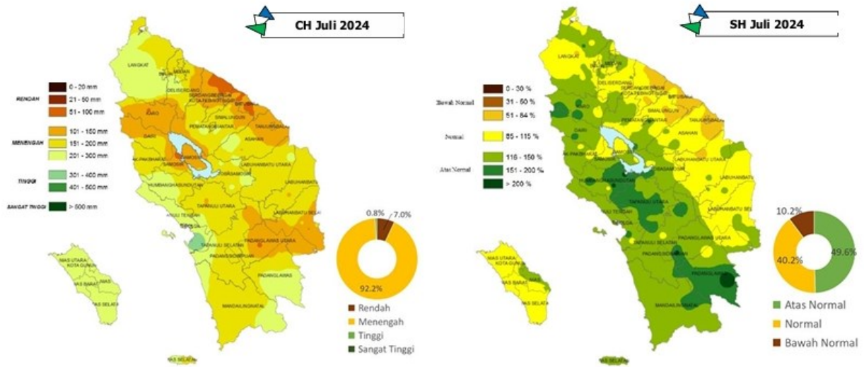
Gambar 2.5.3 Prakiraan Curah Hujan dan Sifat Hujan Juli 2024
