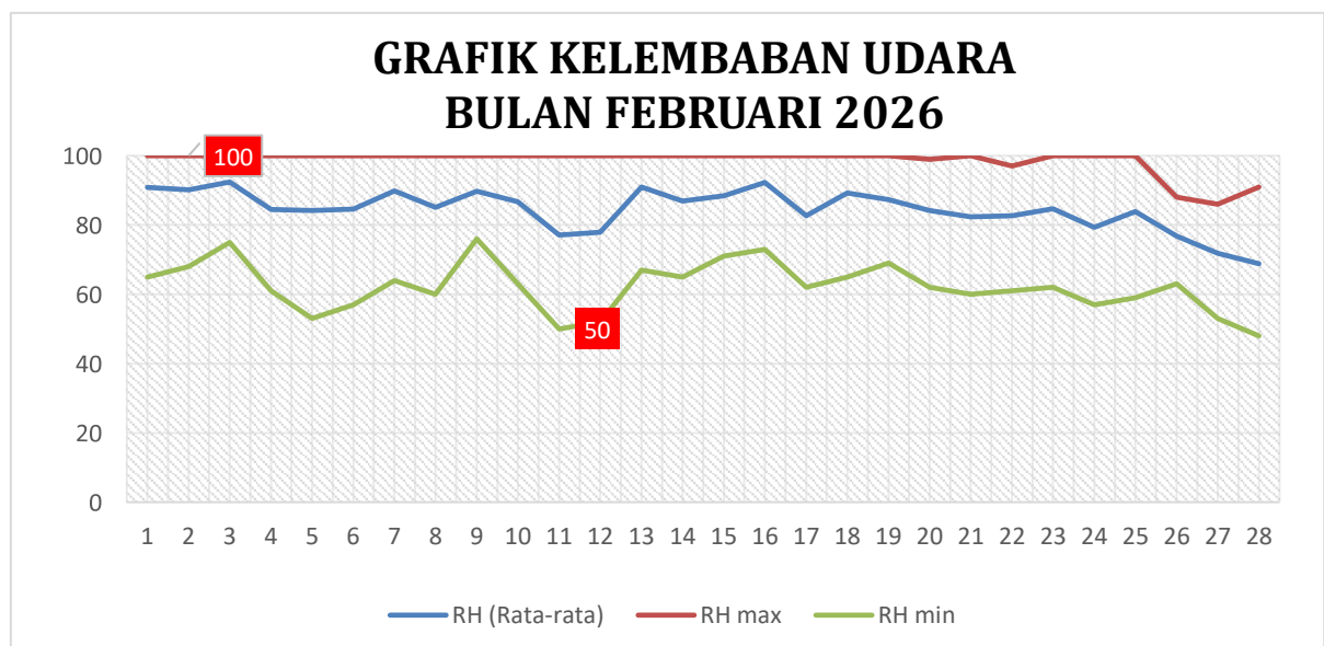
Gambar 2.1.5.1 Grafik Kelembaban Udara Bulan Februari 2026
