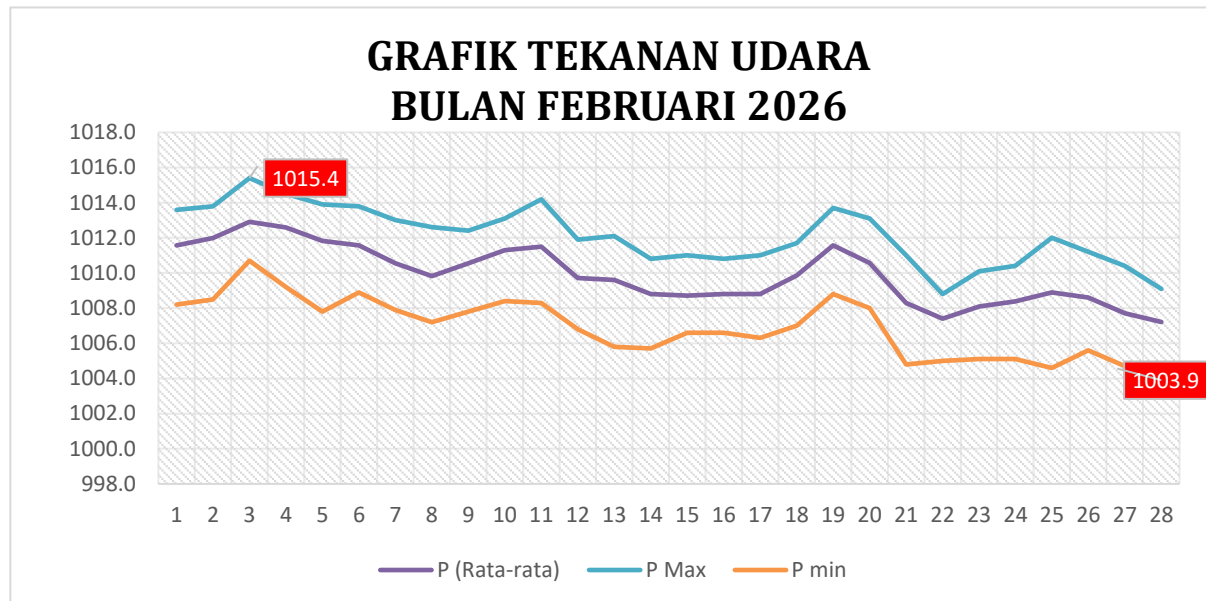
Gambar 2.1.4.1 Grafik Tekanan Udara Bulan Februari 2026
