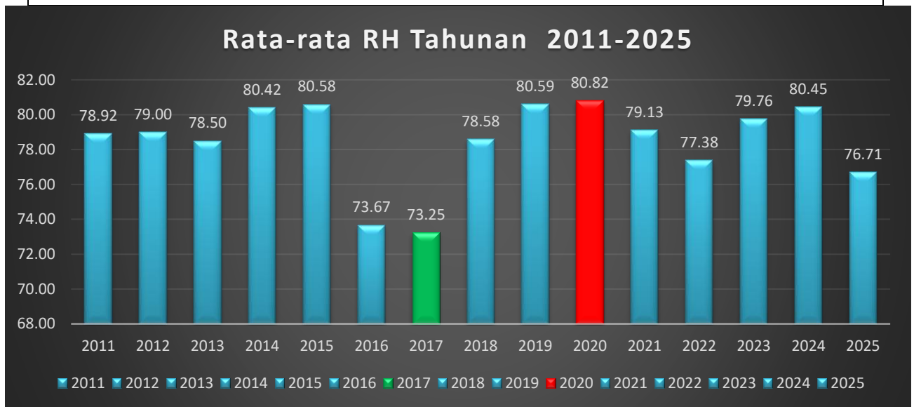
Rata- Rata RH Tahunan 2011-2025 (%)
