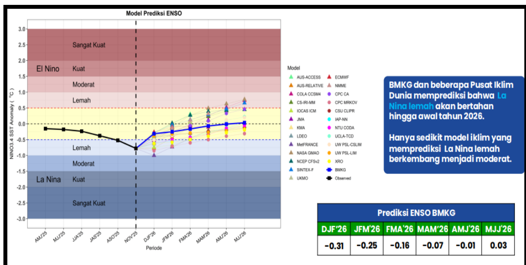
Gambar. 2.2.2 Prediksi ENSO
