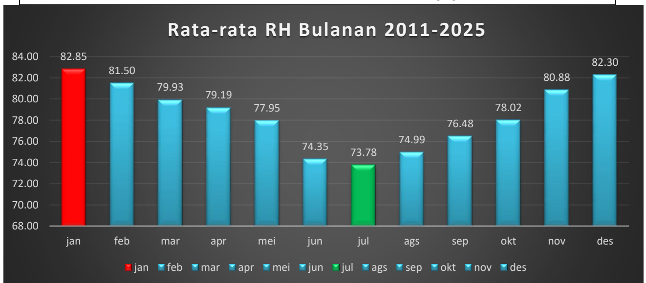
Rata- Rata RH Bulanan 2011-2025 (%)
