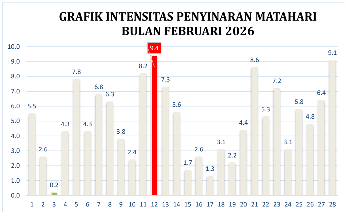
Gambar 2.1.2.1 Grafik Durasi Penyinaran Matahari Bulan Februari 2026
