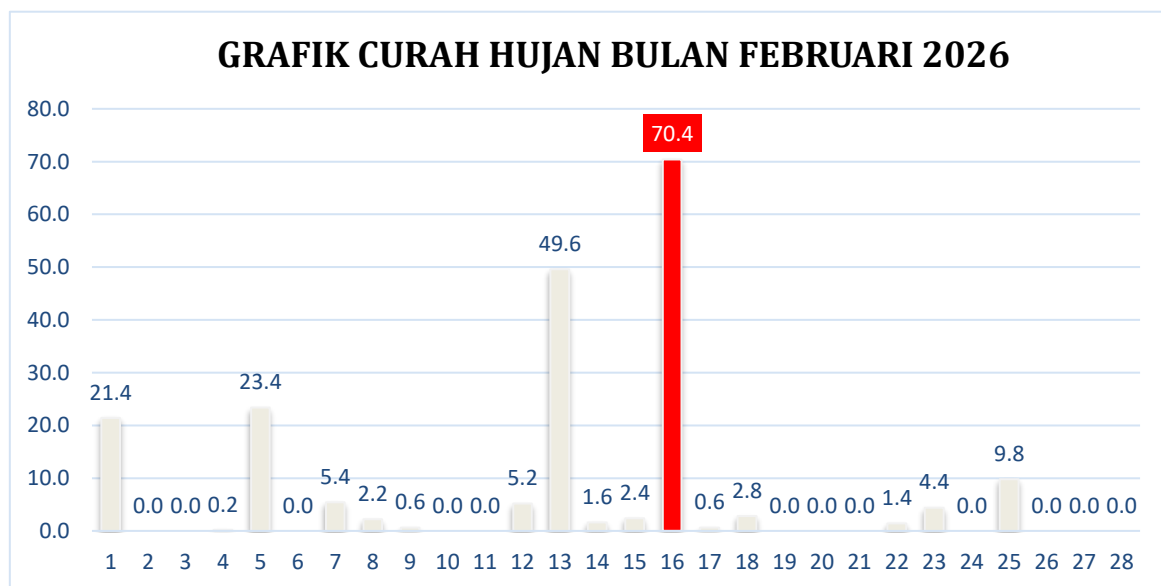
Gambar 2.1.3.2 Intensitas Curah Hujan Bulan Februari 2026
