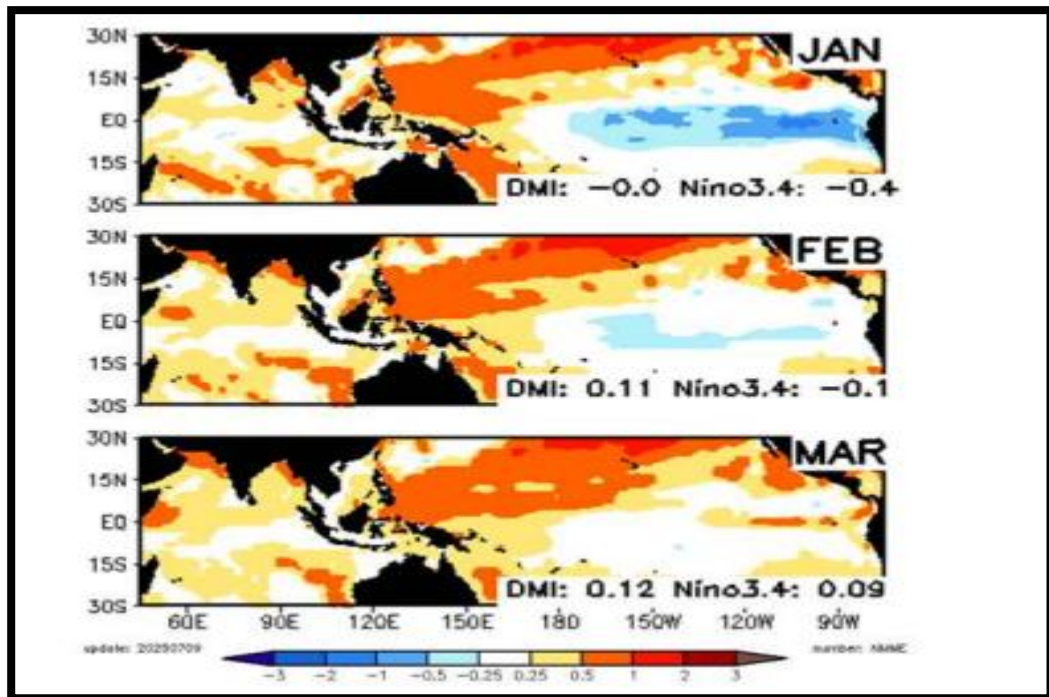
Gambar. 2.2.1 Prediksi Anomali SST
