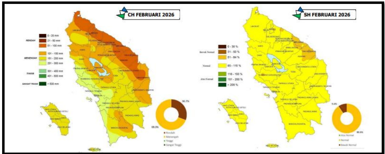
Gambar 2.5.2 Prakiraan Curah Hujan dan Sifat Hujan Februari 2026
