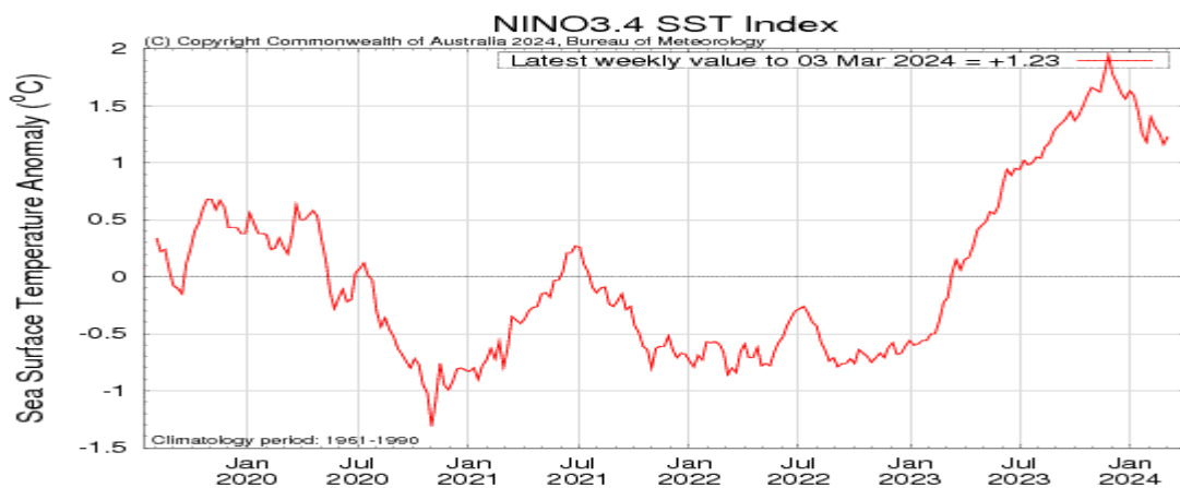
Gambar. 1.2.1 Indeks NINO 3.4 Bulan Pebruari 2024
