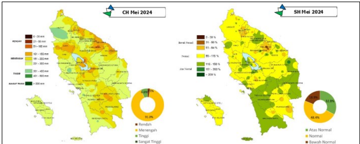
Gambar 2.5.3 Prakiraan Curah Hujan dan Sifat Hujan Mei 2024
