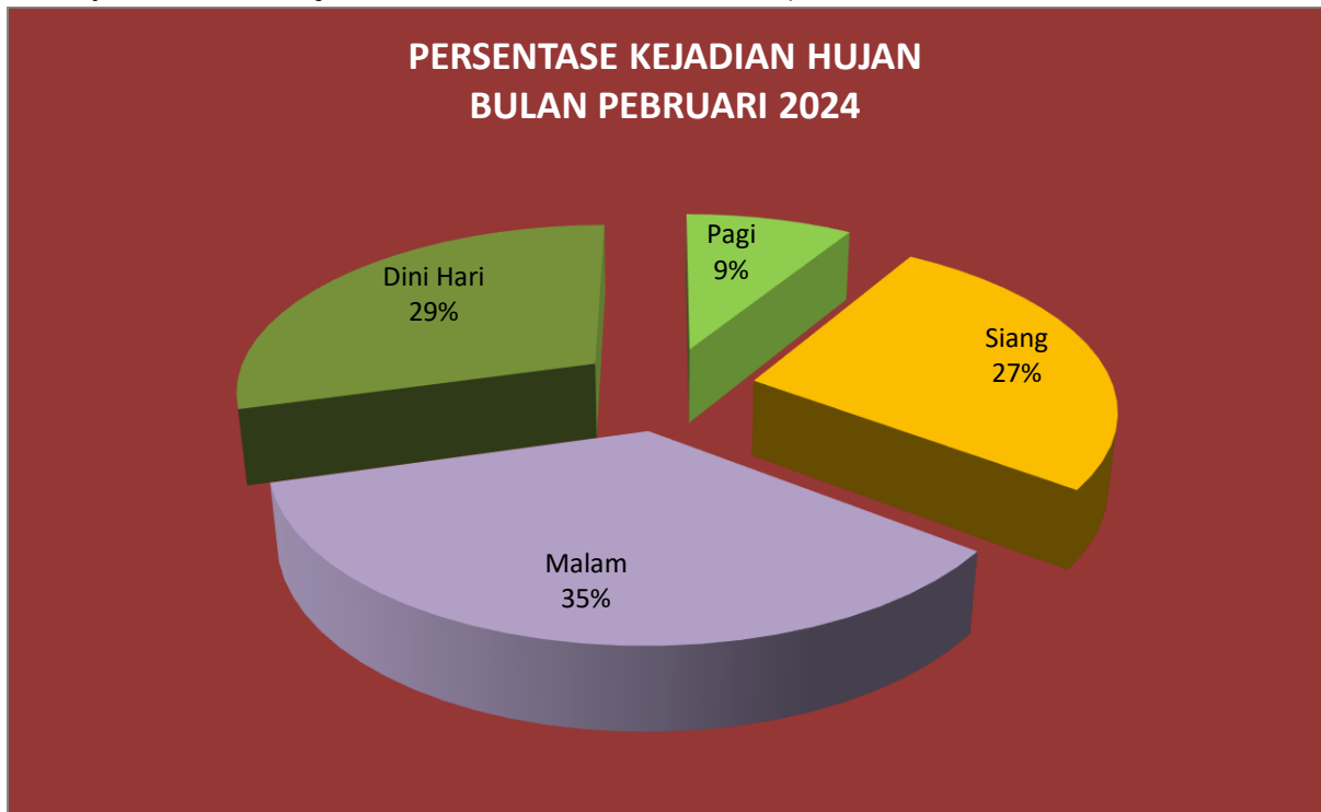
Gambar 2.1.3.1 Persentase Kejadian Hujan Bulan Pebruari 2024
