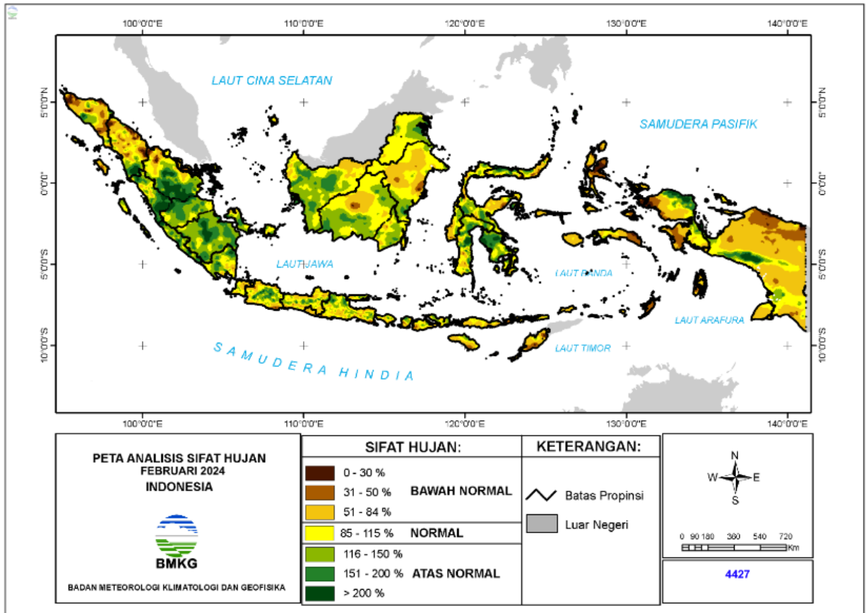
Gambar 1.2.4 Peta Analisis Curah Hujan dan Sifat Hujan Bulan Pebruari 2024
