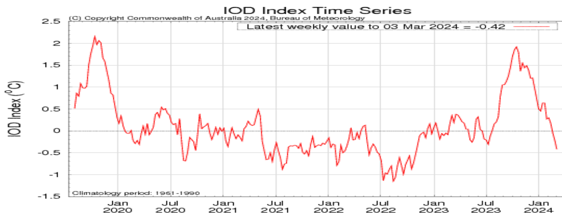
Gambar. 1.2.2 Indeks IOD Bulan Pebruari 2024
