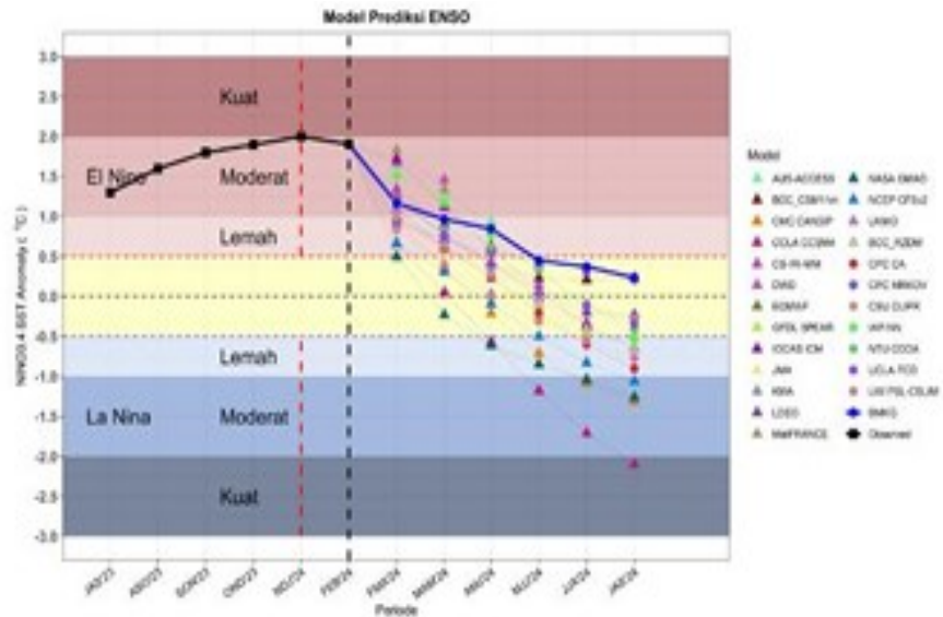
Gambar. 2.2.2 Prediksi ENSO
