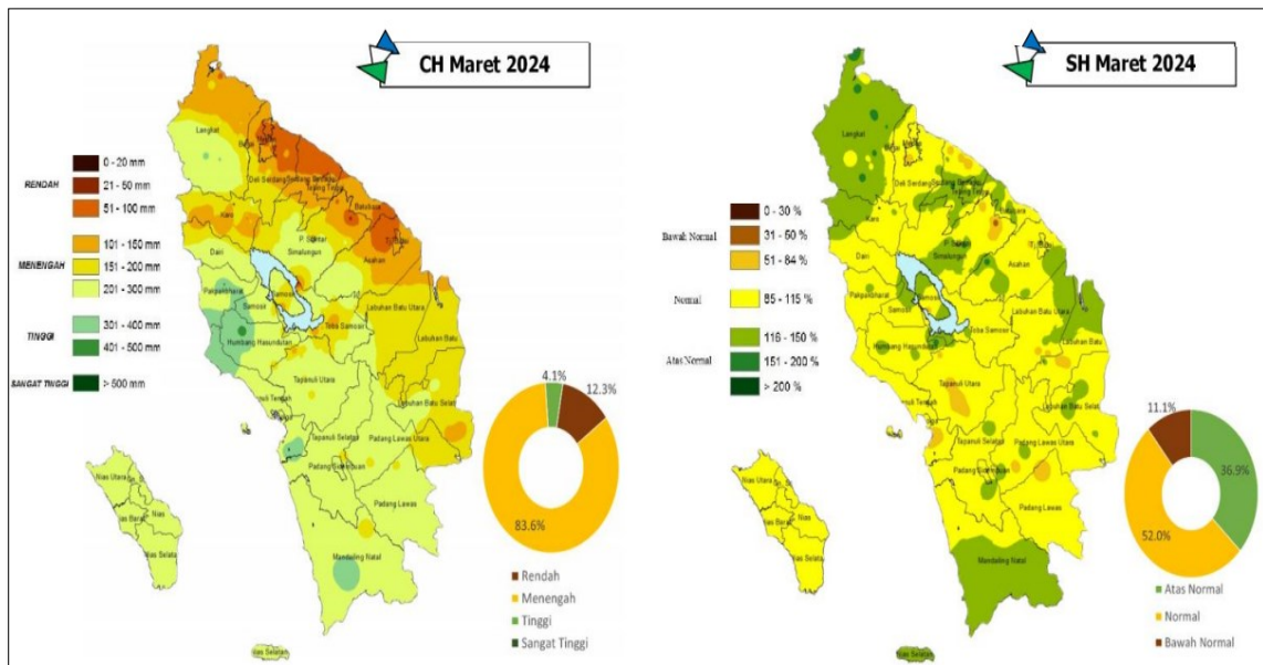
Gambar 2.5.1 Prakiraan Curah Hujan dan Sifat Hujan Maret 2024
