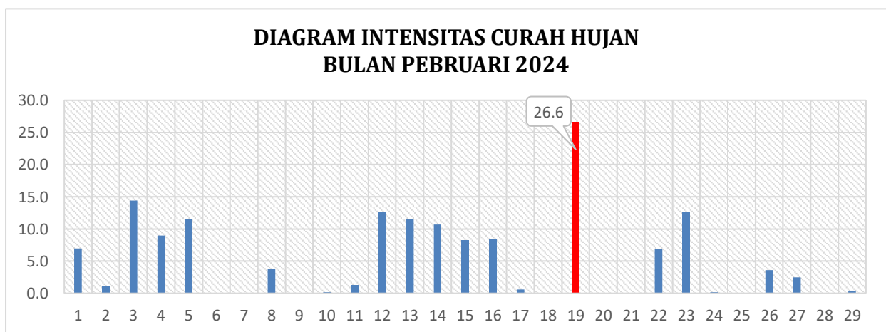
Gambar 2.1.3.2 Intensitas Curah Hujan Bulan Pebruari 2024
