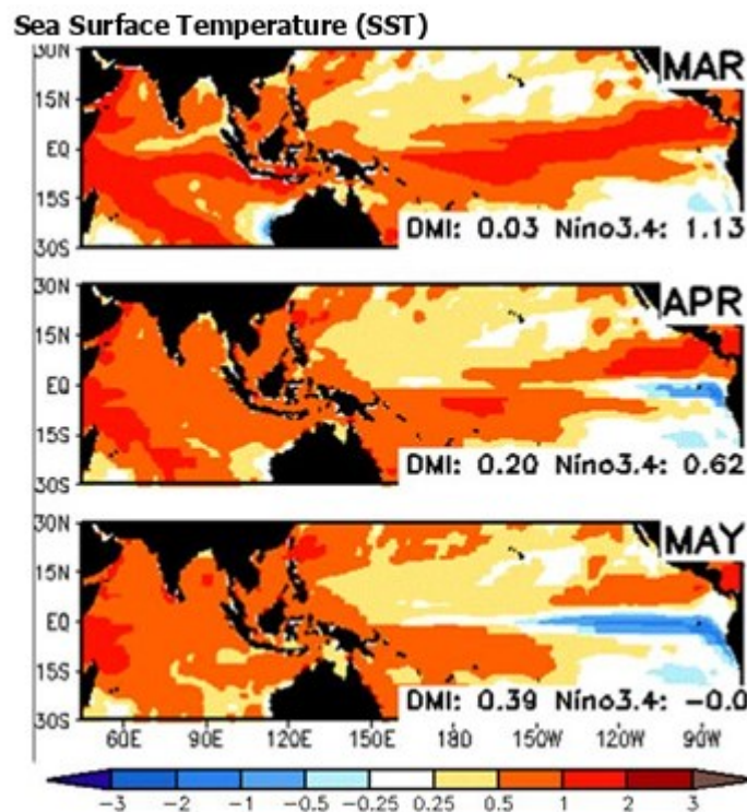
Gambar. 2.2.1 Prediksi Anomali SST
