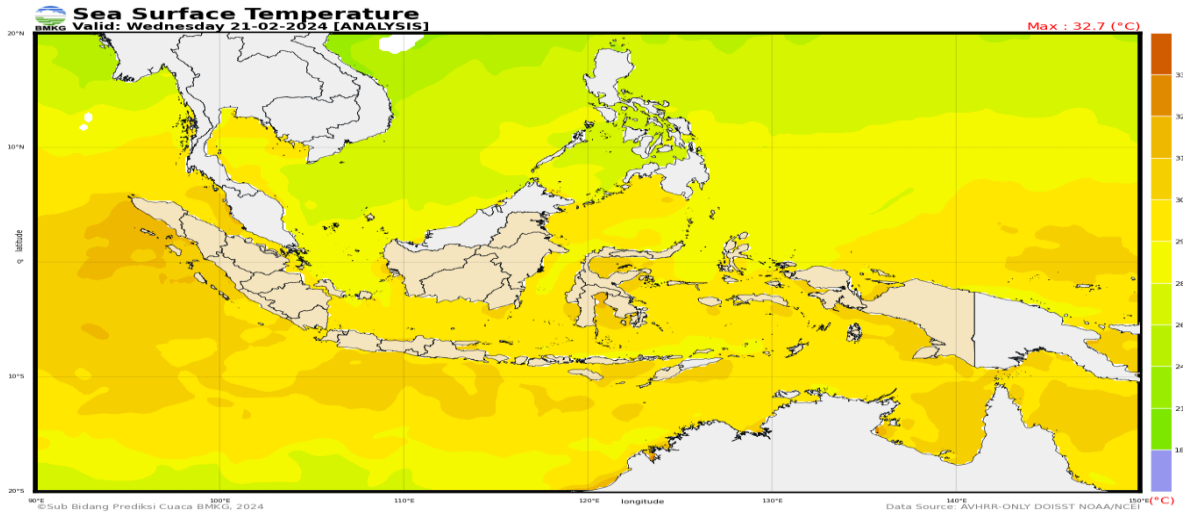
Gambar 1.2.3 SST Bulan Pebruari 2024
