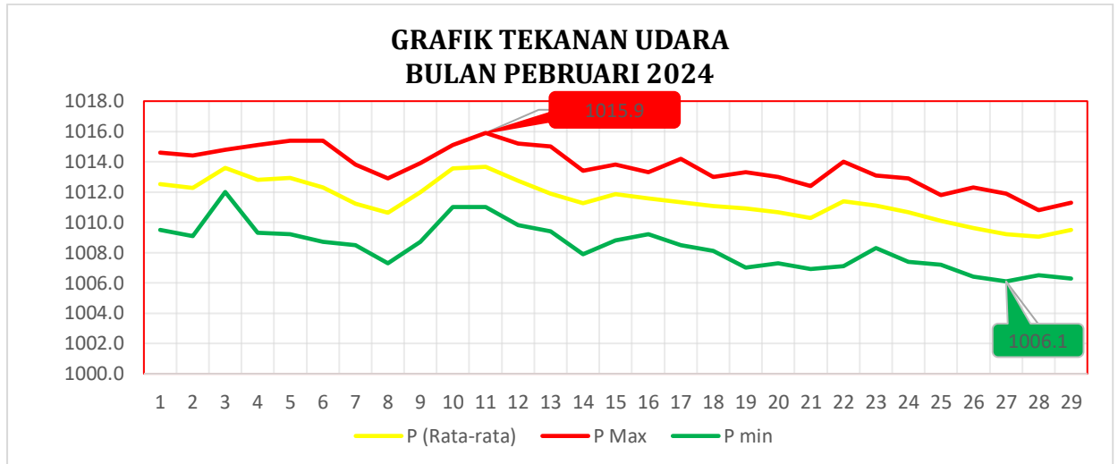
Gambar 2.1.4.1 Grafik Tekanan Udara Bulan Pebruari 2024
