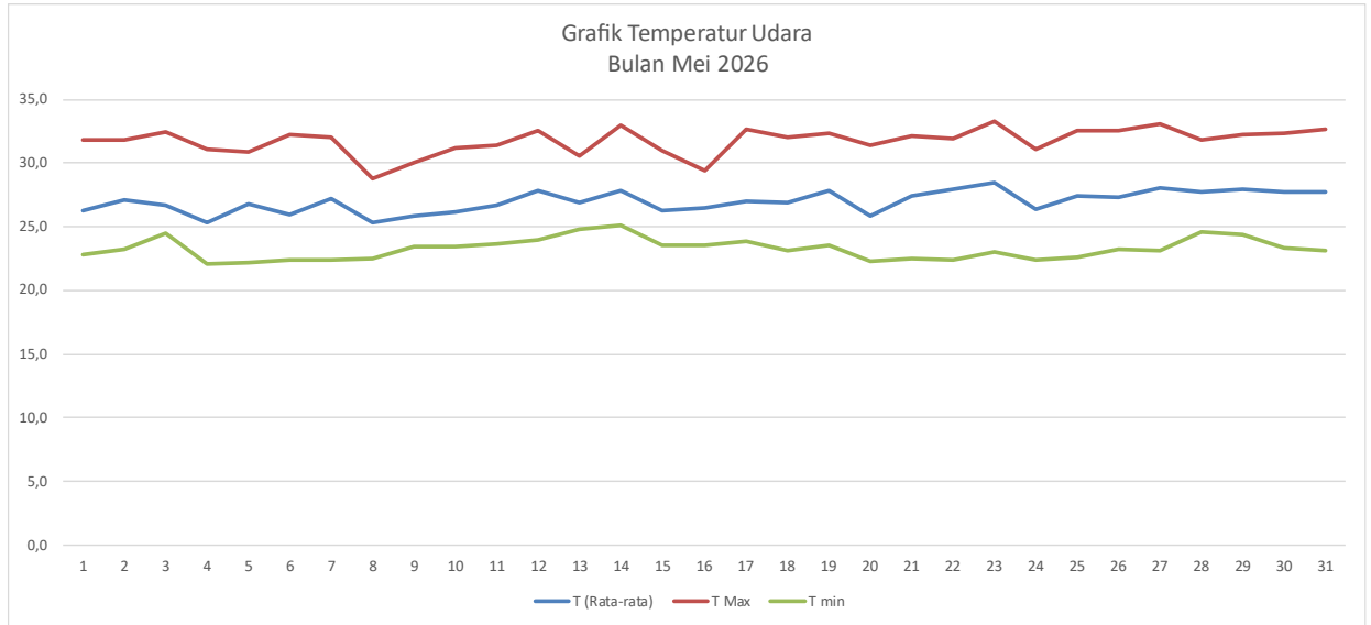
Gambar 2.1.1.1 Grafik Suhu Udara Bulan Mei 2026
