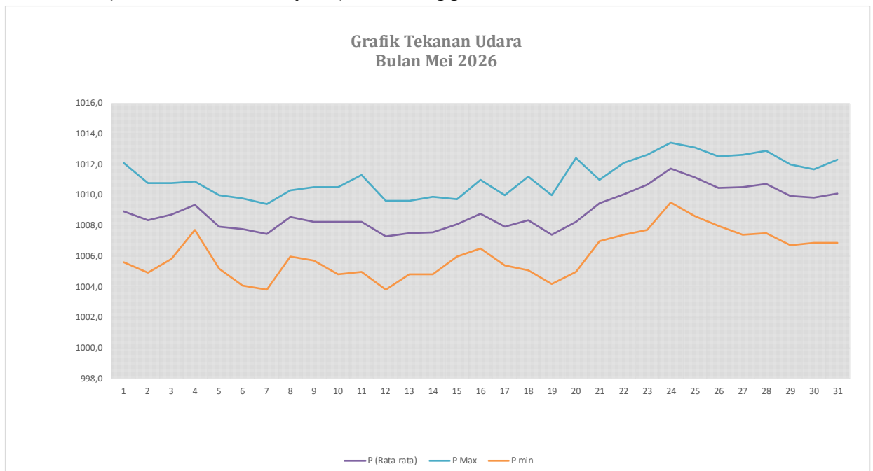
Gambar 2.1.4.1 Grafik Tekanan Udara Bulan Mei 2026
