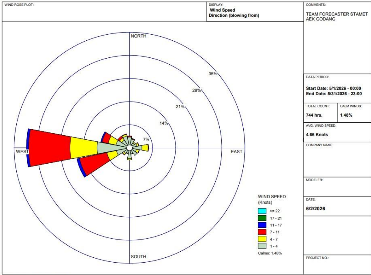
Gambar 2.1.6.1 Grafik Angin Bulan Mei 2026
