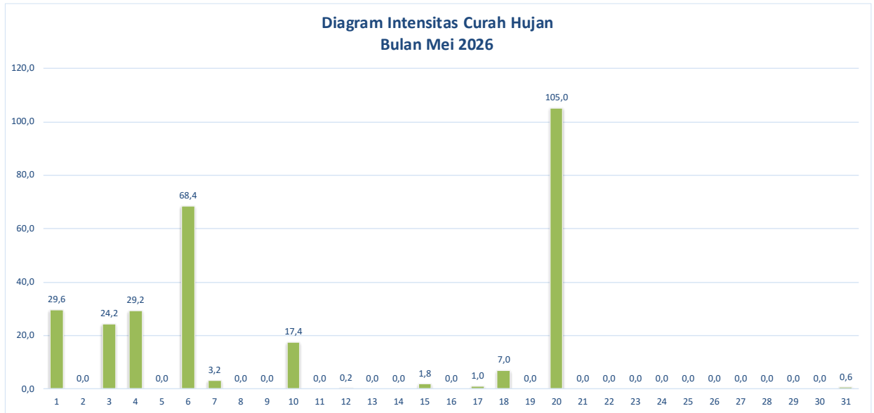
Gambar 2.1.3.1 Intensitas Curah Hujan Bulan Mei 2026
