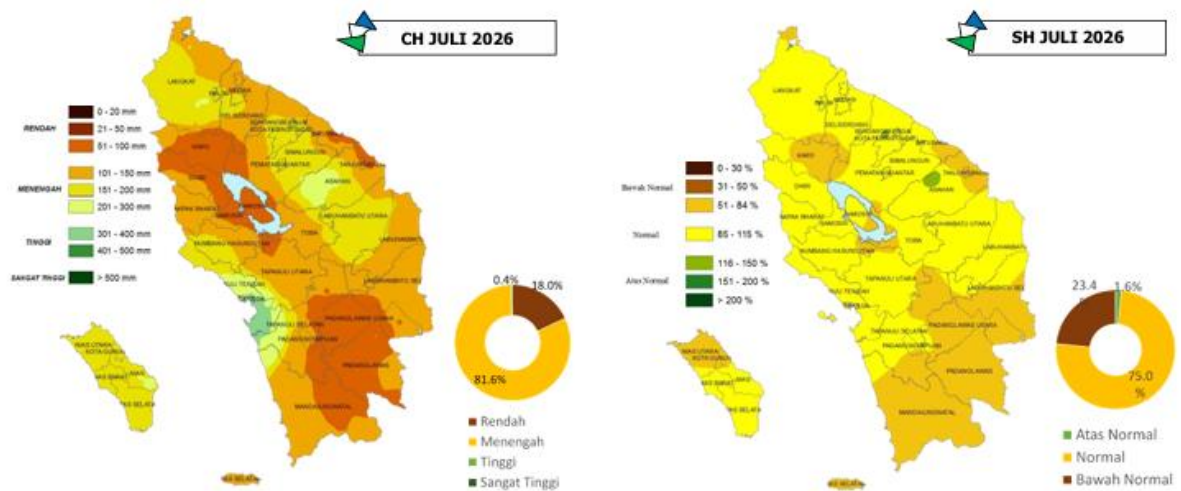
Sumber BMKG Gambar 2.5.2 Prakiraan Curah Hujan dan Sifat Hujan Juli 2026
