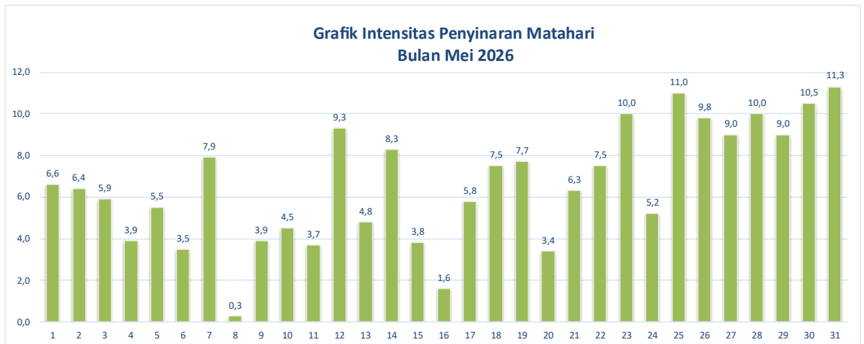
Gambar 2.1.2.1 Grafik Durasi Penyinaran Matahari Bulan Mei 2026
