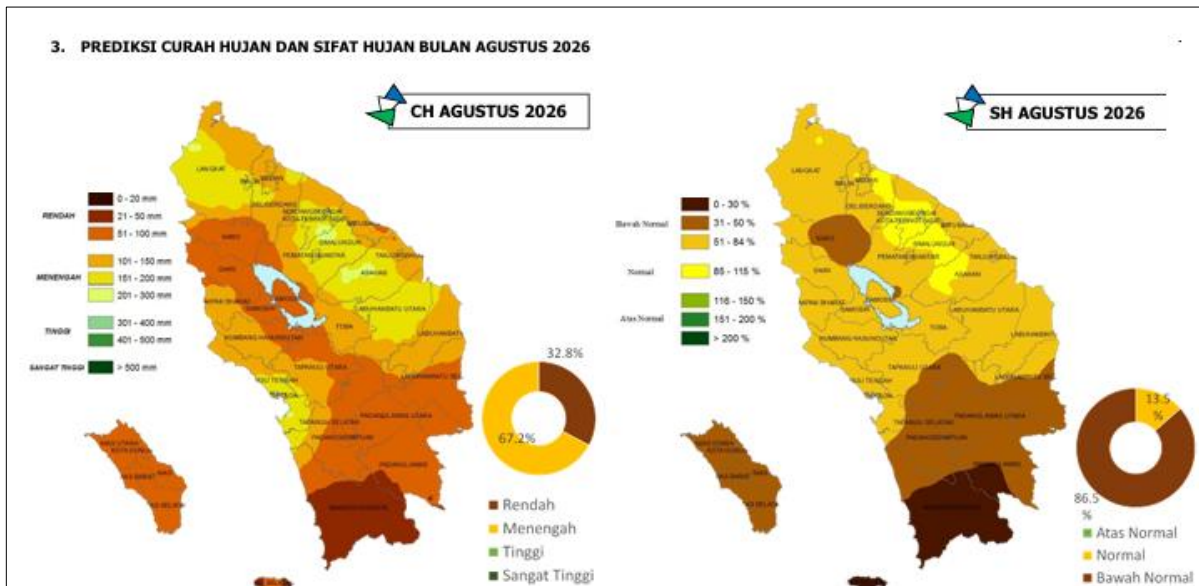
Sumber BMKG Gambar 2.5.3 Prakiraan Curah Hujan dan Sifat Hujan Agustus 2026
