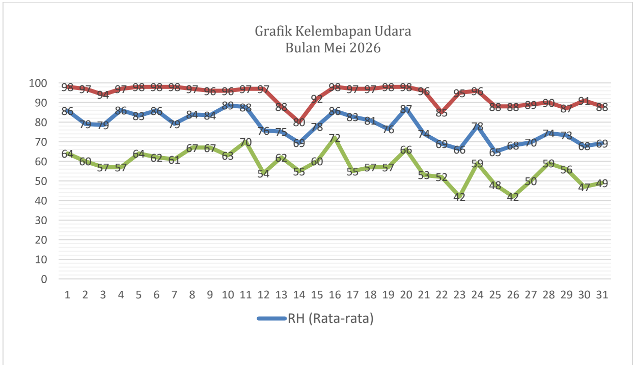
Gambar 2.1.5.1 Grafik Kelembaban Udara Bulan Mei 2026
