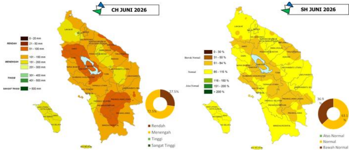
Sumber BMKG Gambar 2.5.1 Prakiraan Curah Hujan dan Sifat Hujan Juni 2026
