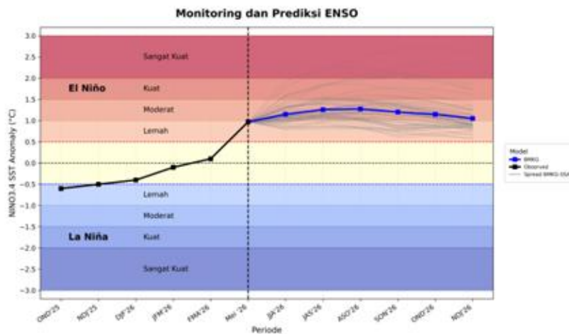
Sumber BMKG Gambar. 2.2.2 Prediksi ENSO
