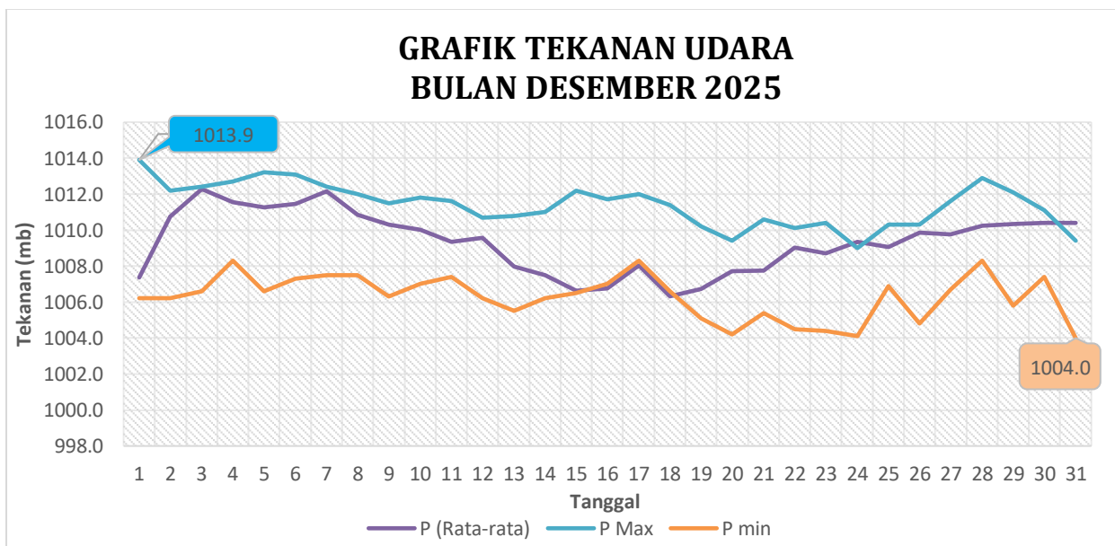
Gambar 2.1.4.1 Grafik Tekanan Udara Bulan Desember 2025
