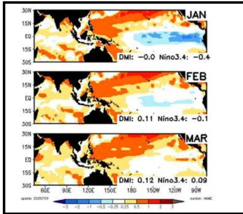
Gambar. 2.2.1 Prediksi Anomali SST
