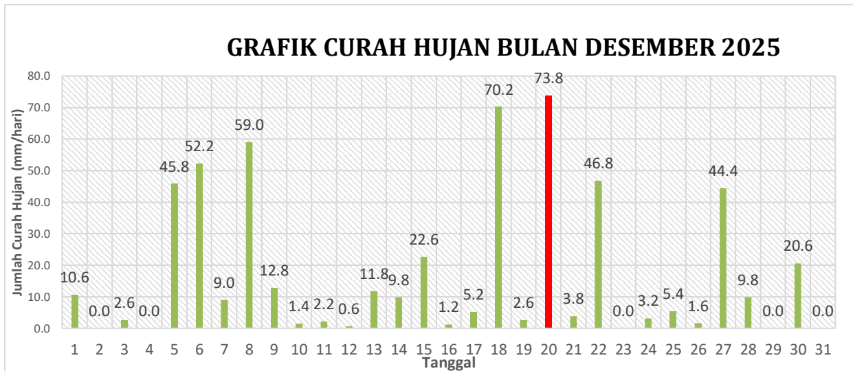
Gambar 2.1.3.2 Intensitas Curah Hujan Bulan Desember 2025
