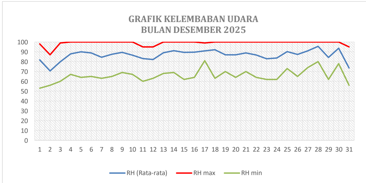
Gambar 2.1.5.1 Grafik Kelembaban Udara Bulan Desember 2025
