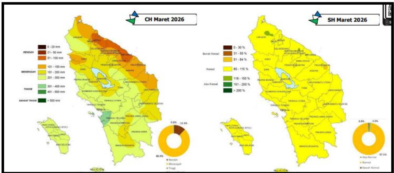
Gambar 2.5.3 Prakiraan Curah Hujan dan Sifat Hujan Maret 2026
