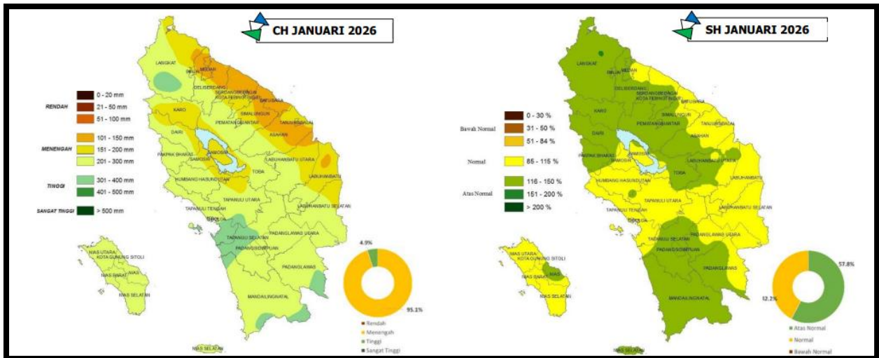
Gambar 2.5.1 Prakiraan Curah Hujan dan Sifat Hujan Januari 2026
