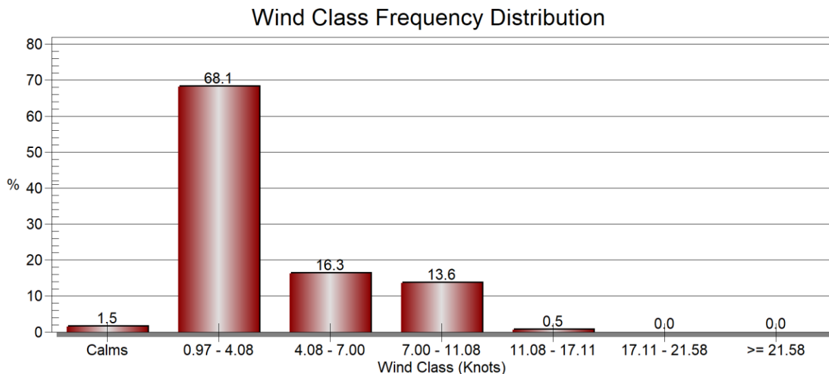
Gambar 2.1.6.1 Grafik Angin Bulan Desember 2025
