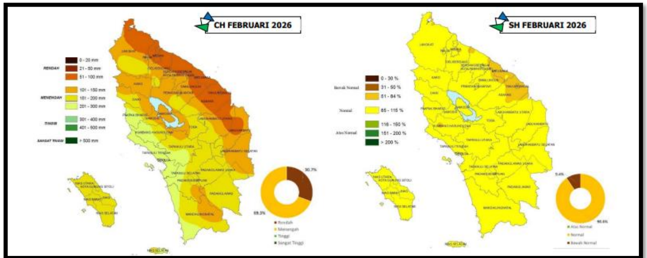
Gambar 2.5.2 Prakiraan Curah Hujan dan Sifat Hujan Pebruari 2026
