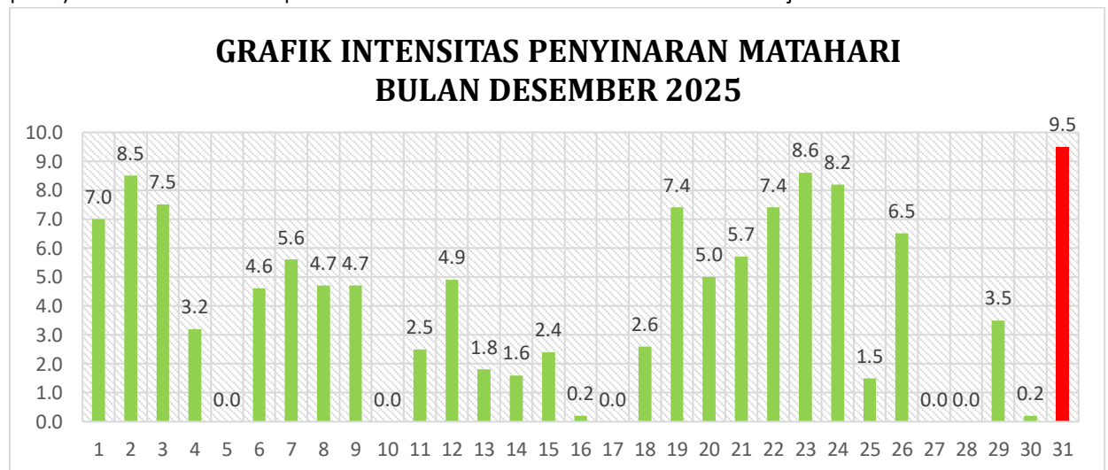
Gambar 2.1.2.1 Grafik Durasi Penyinaran Matahari Bulan Desember 2025
