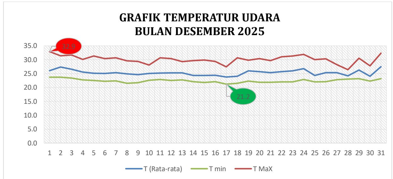
Gambar 2.1.1.1 Grafik Suhu Udara Bulan Desember 2025
