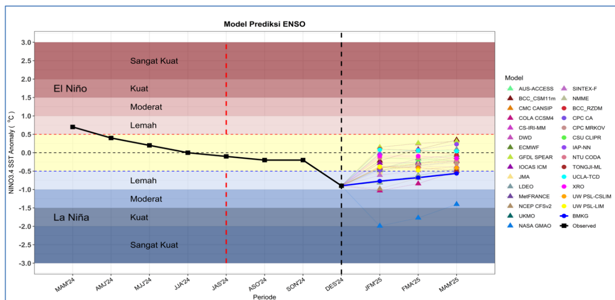
Gambar. 2.2.2 Prediksi ENSO
