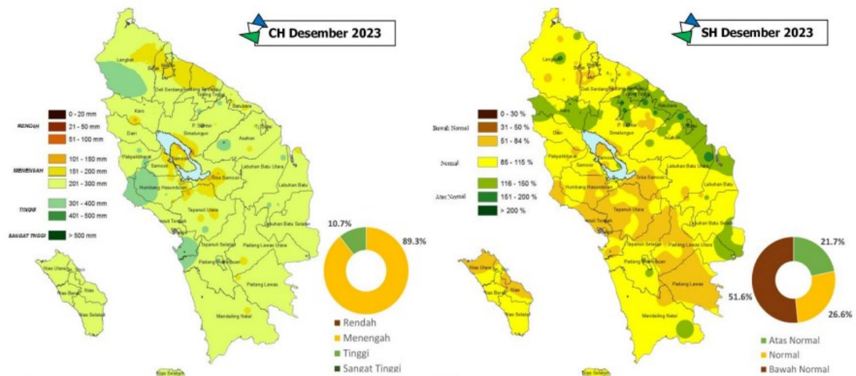
Gambar 2.5.2 Prakiraan Curah Hujan dan Sifat Hujan Desember 2023
