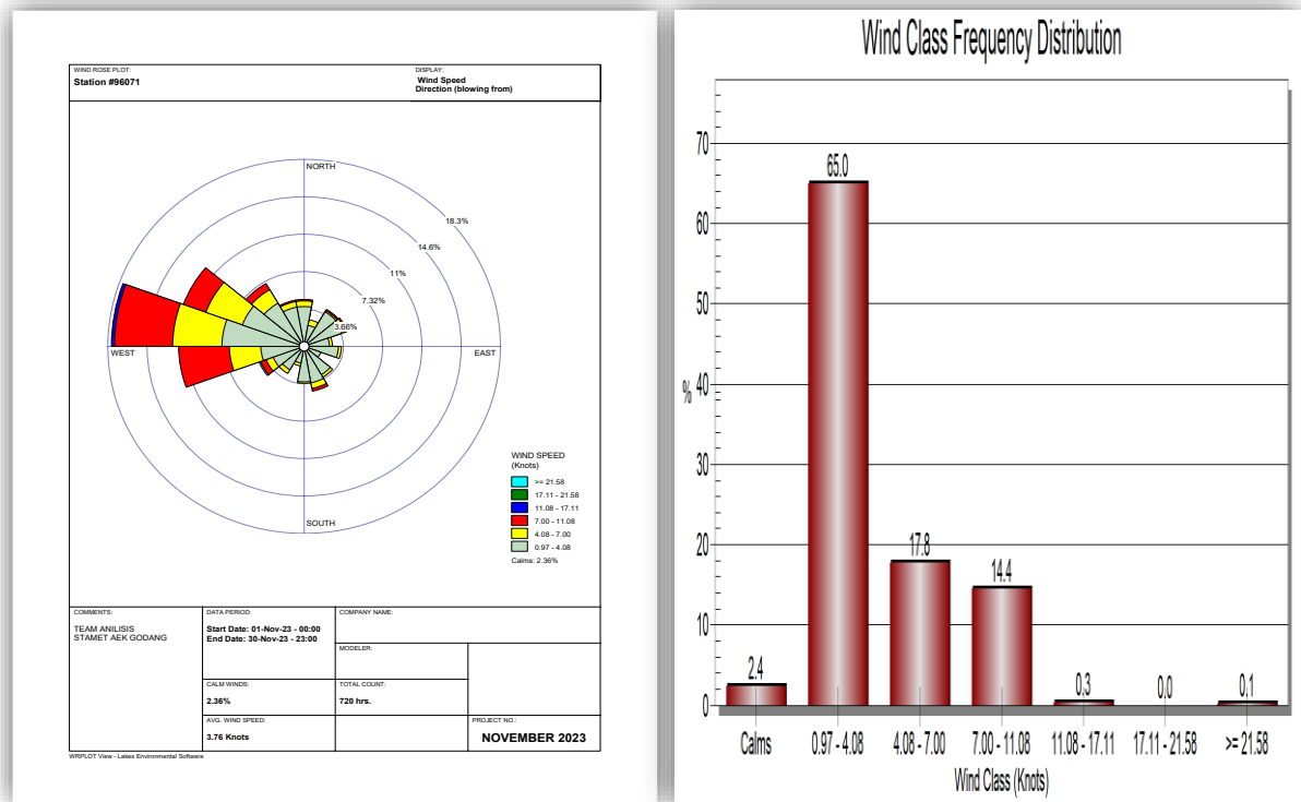
Gambar 2.1.6.1 Diagram Arah dan Kecepatan Angin Bulan November 2023
