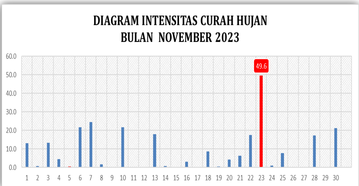
Gambar 2.1.3.2 Intensitas Curah Hujan Bulan November 2023
