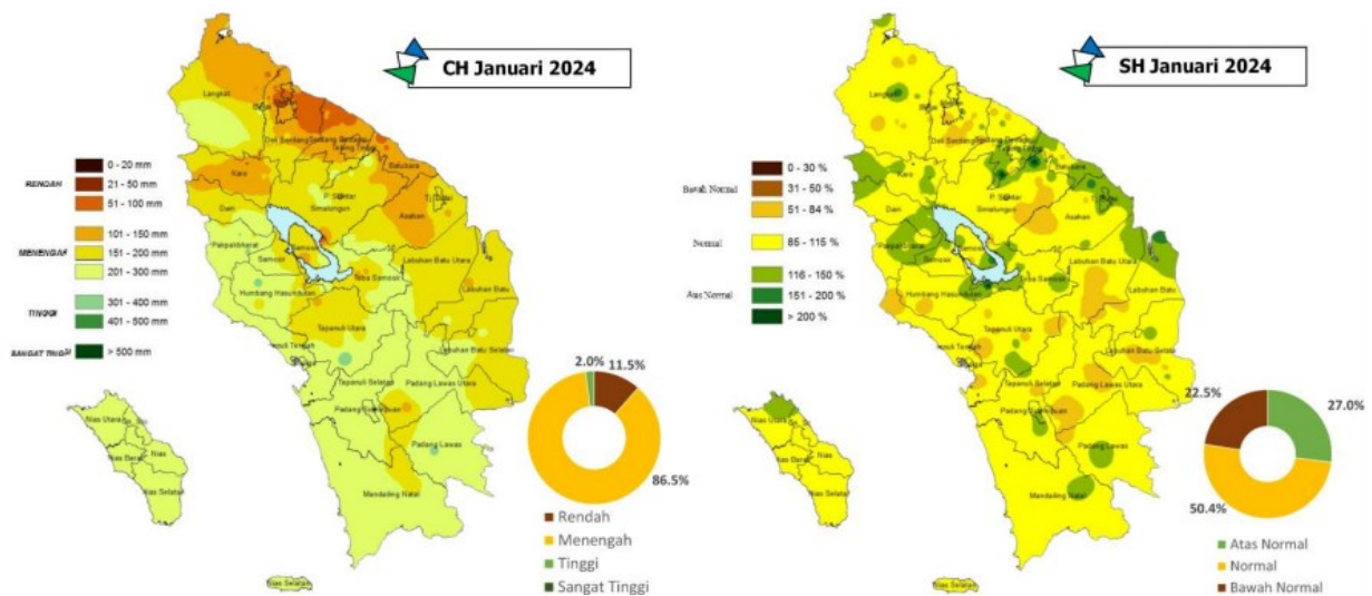
Gambar 2.5.3 Prakiraan Curah Hujan dan Sifat Hujan Januari 2024
