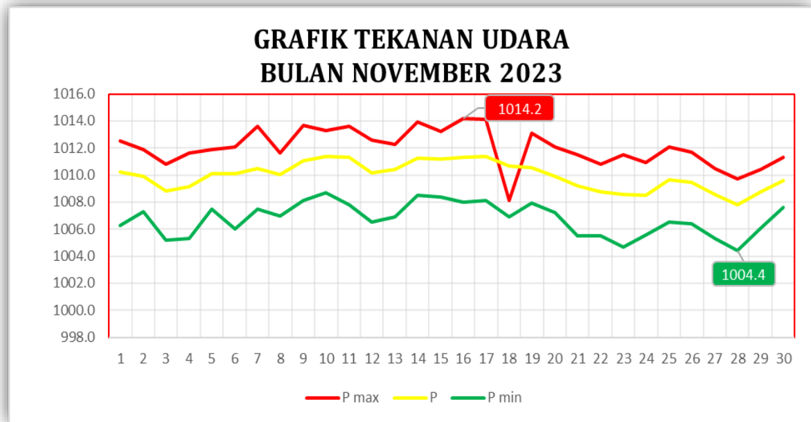
Gambar 2.1.4.1 Grafik Tekanan Udara Bulan November 2023
