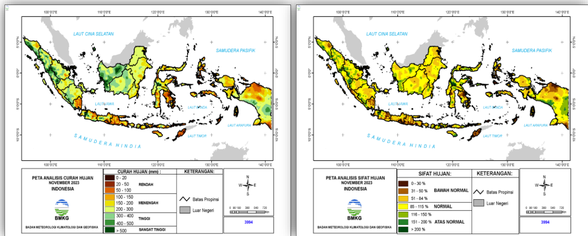
Gambar 1.2.4 Peta Analisis Curah Hujan dan Sifat Hujan Bulan November 2023
