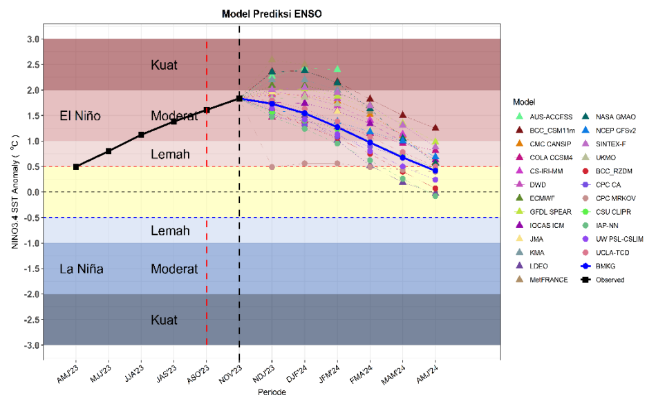
Gambar. 2.2.2 Prediksi ENSO
