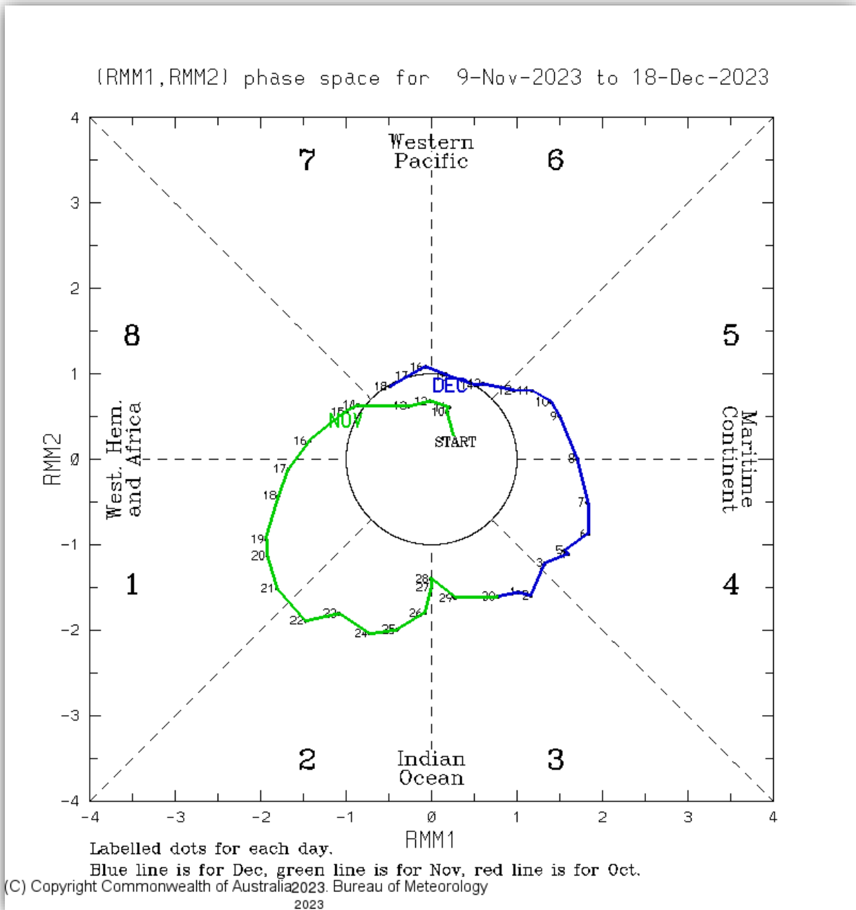
Gambar 1.2.5 Peta MJO Bulan November 2023
