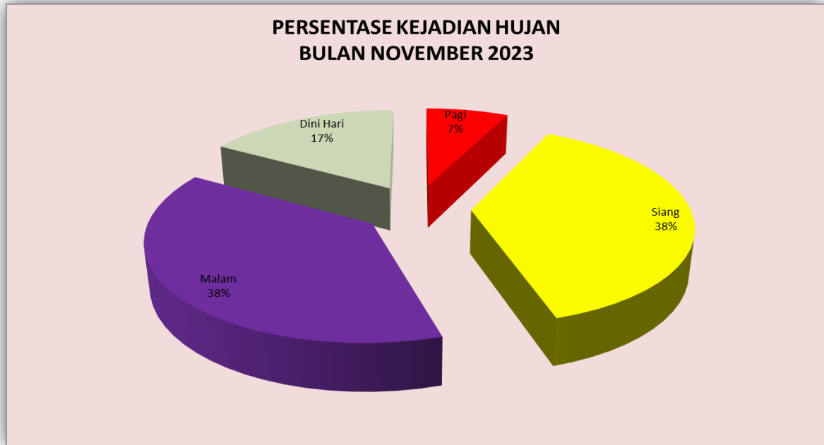
Gambar 2.1.3.1 Persentase Kejadian Hujan Bulan November 2023
