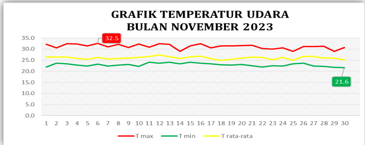
Gambar 2.1.1.1 Grafik Suhu Udara Bulan November 2023
