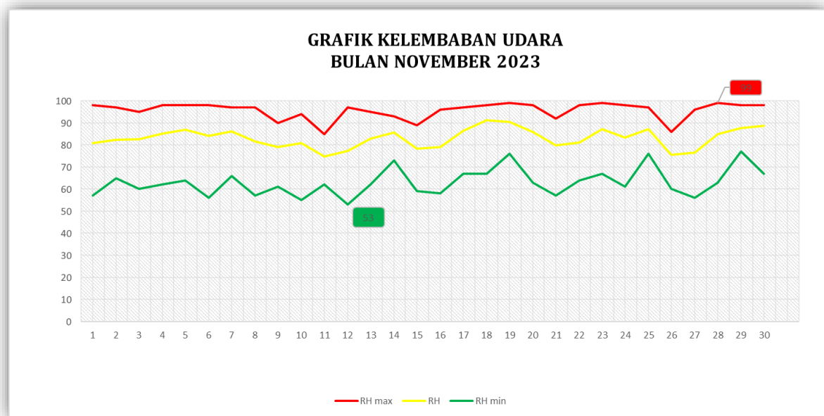
Gambar 2.1.5.1 Grafik Kelembaban Udara Bulan November 2023
