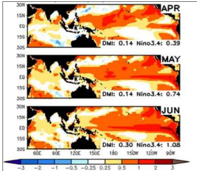
Gambar. 2.2.1 Prediksi Anomali SST
