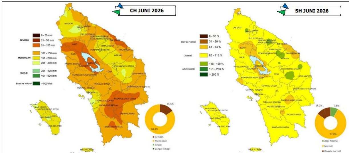
Gambar 2.5.3 Prakiraan Curah Hujan dan Sifat Hujan Juni 2026
