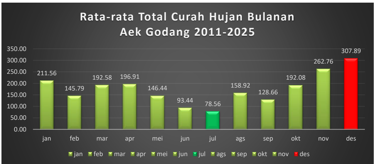
Gambar 3.1.3 Grafik Rata-Rata Curah Hujan
