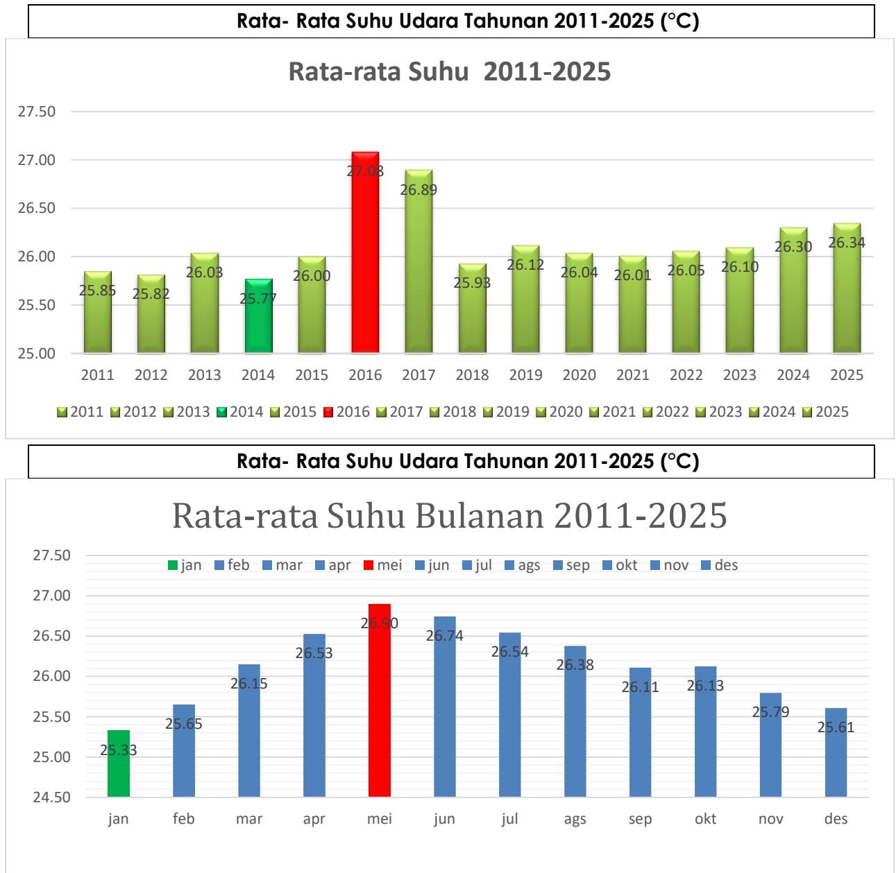
Gambar 3.1.2 Grafik Rata-Rata Suhu Udara
