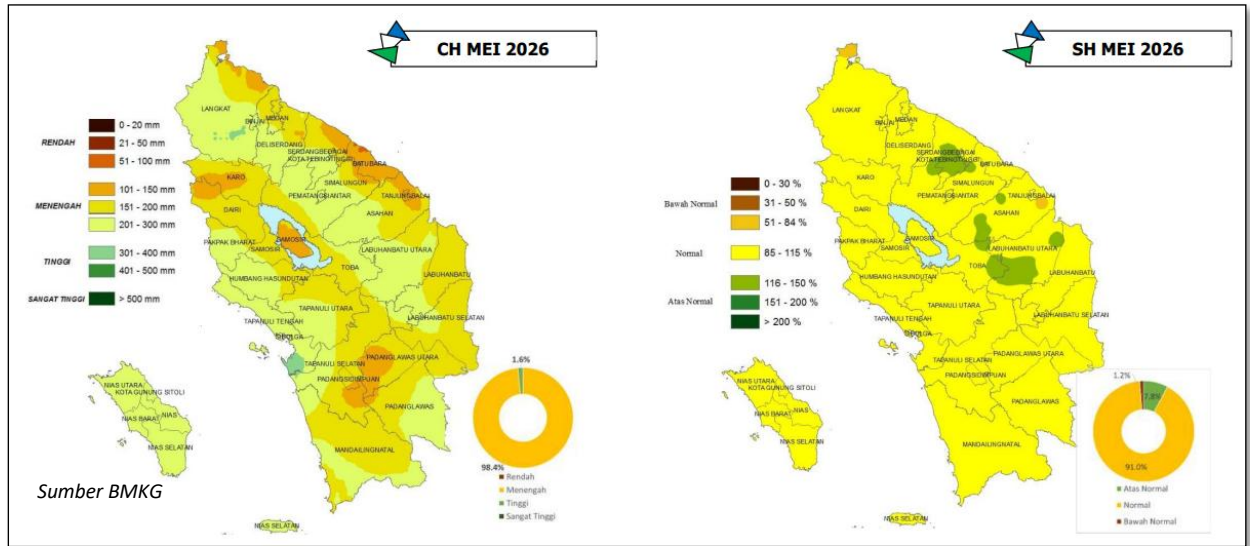
Gambar 2.5.2 Prakiraan Curah Hujan dan Sifat Hujan Mei 2026
