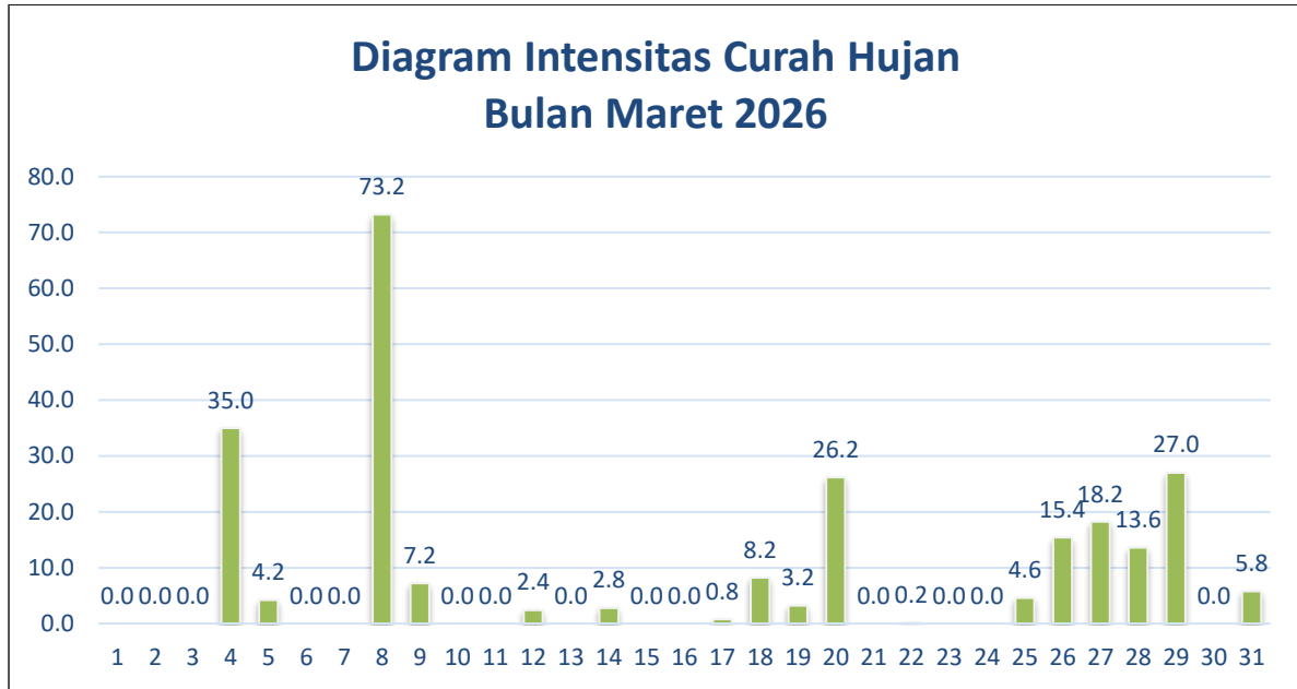
Gambar 2.1.3.1 Intensitas Curah Hujan Bulan Maret 2026
