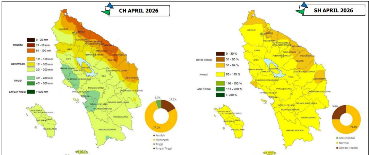
Gambar 2.5.1 Prakiraan Curah Hujan dan Sifat Hujan April 2026
