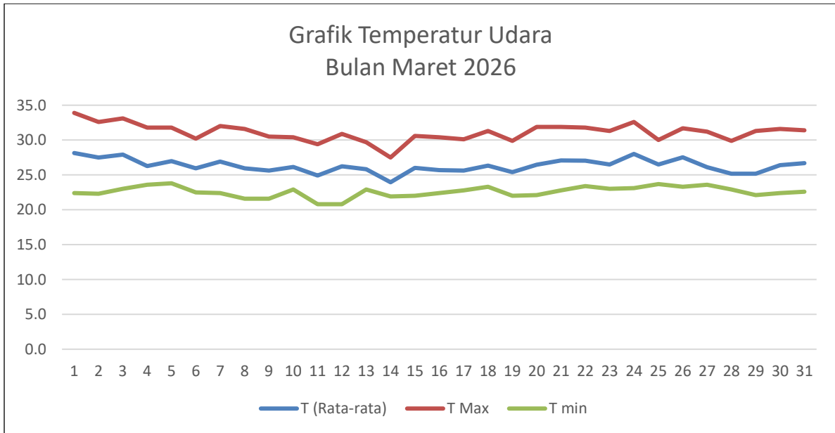
Gambar 2.1.1.1 Grafik Suhu Udara Bulan Maret 2026
