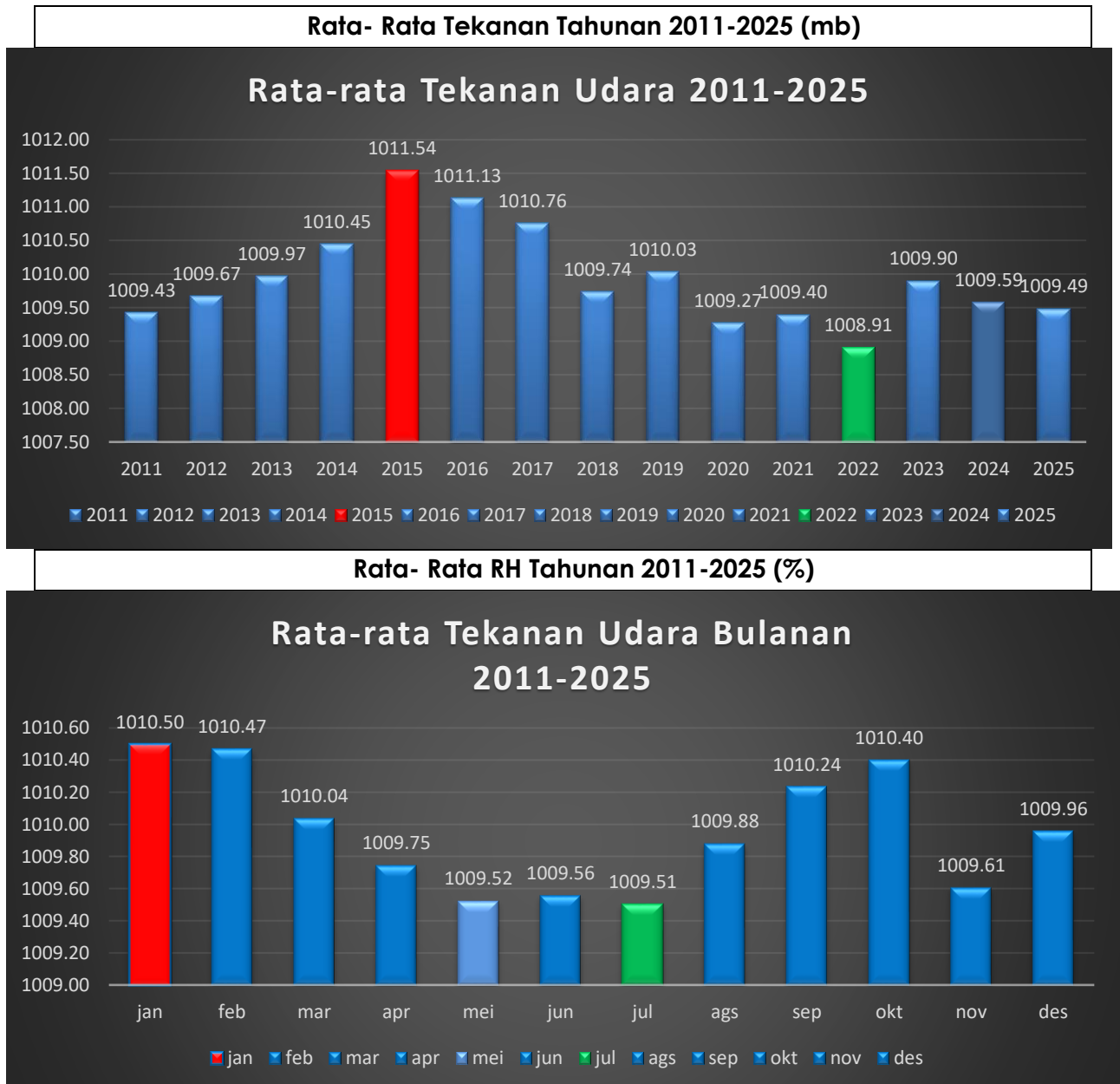
Gambar 3.1.5 Grafik Rata-Rata Tekanan
