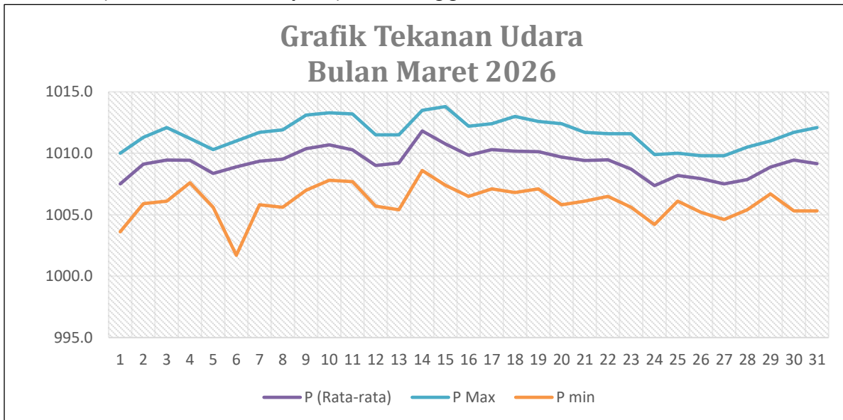
Gambar 2.1.4.1 Grafik Tekanan Udara Bulan Maret 2026
