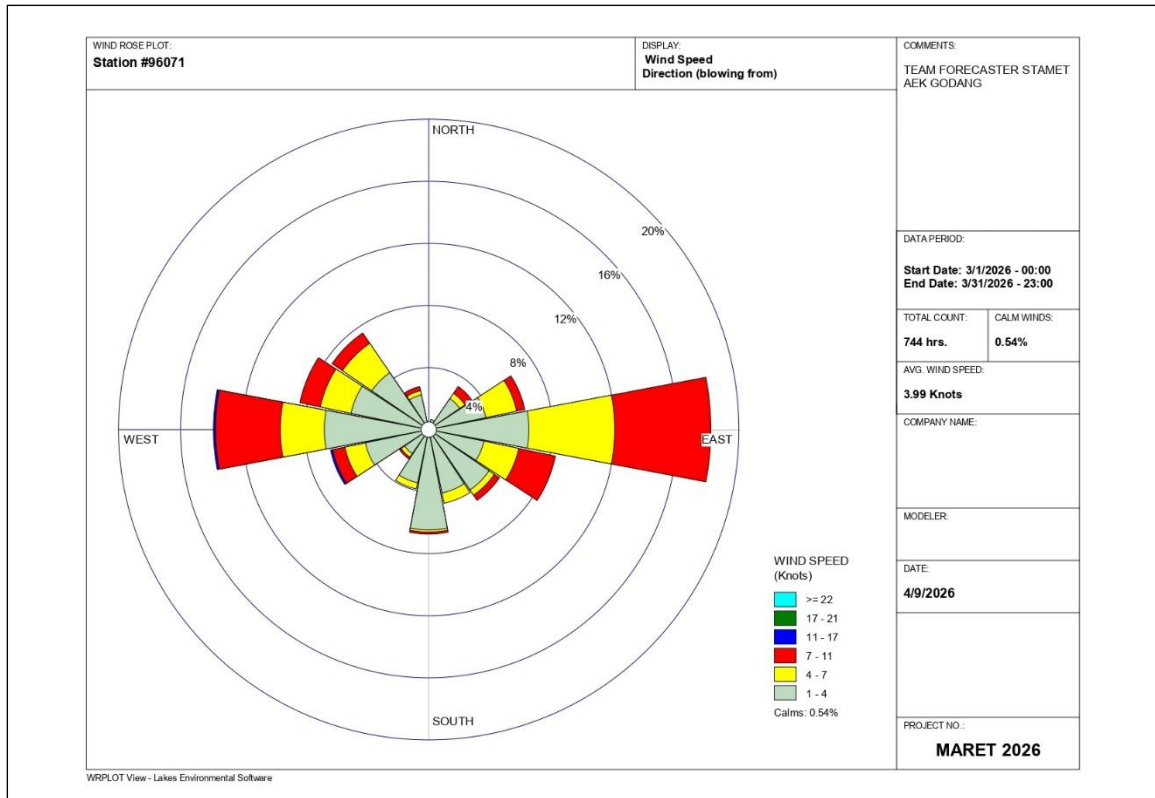
Gambar 2.1.6.1 Grafik Angin Bulan Maret 2026
