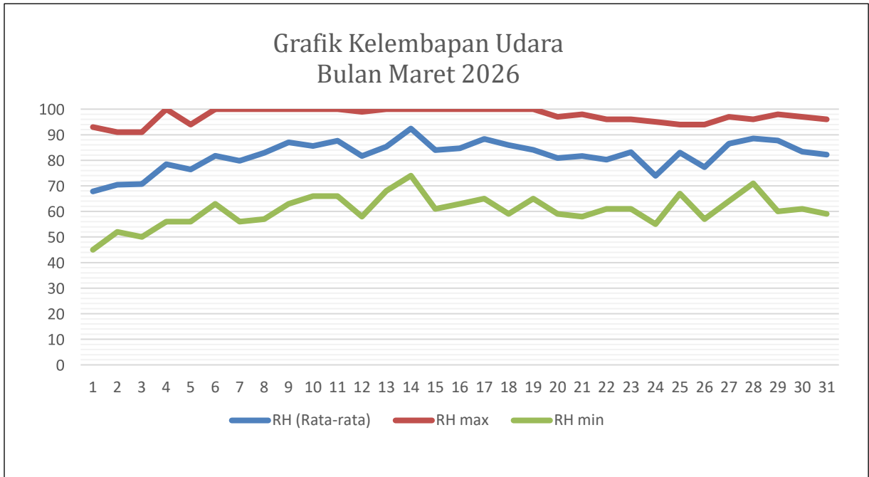
Gambar 2.1.5.1 Grafik Kelembaban Udara Bulan Maret 2026
