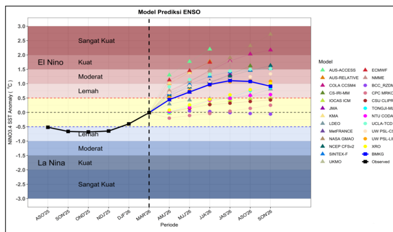
Gambar. 2.2.2 Prediksi ENSO
