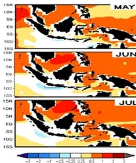
Gambar. 2.2.1 Prediksi Anomali SST
