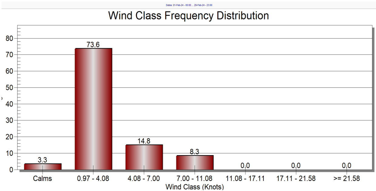
Gambar 2.1.6.1 Diagram Arah dan Kecepatan Angin Bulan Maret 2024
