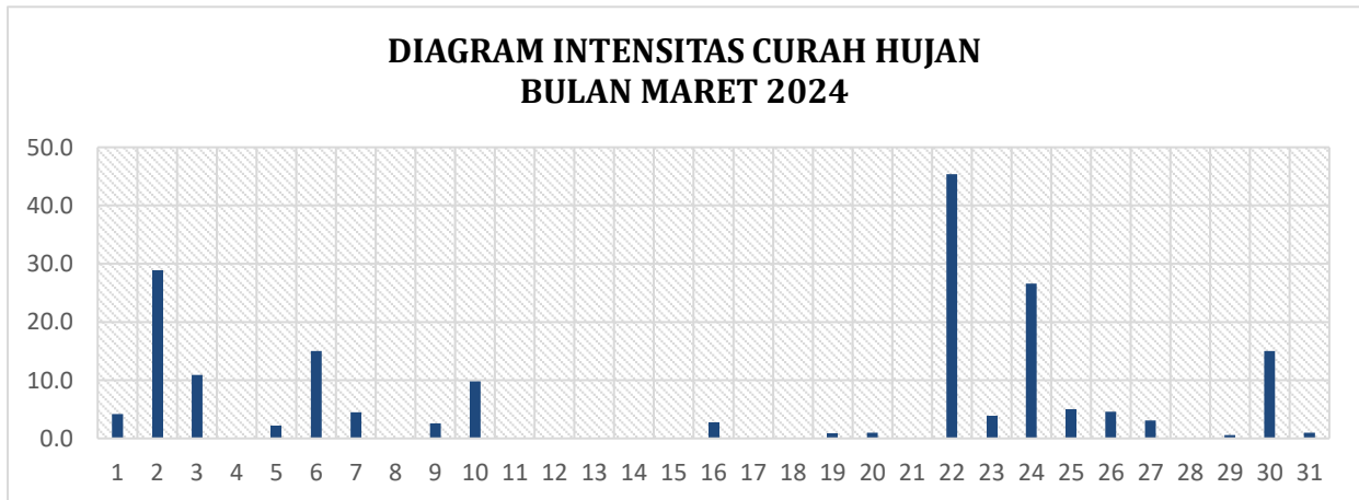
Gambar 2.1.3.2 Intensitas Curah Hujan Bulan Maret 2024
