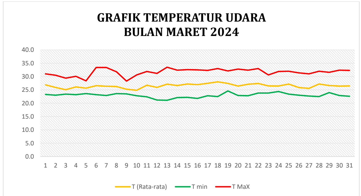
Gambar 2.1.1.1 Grafik Suhu Udara Bulan Maret 2024
