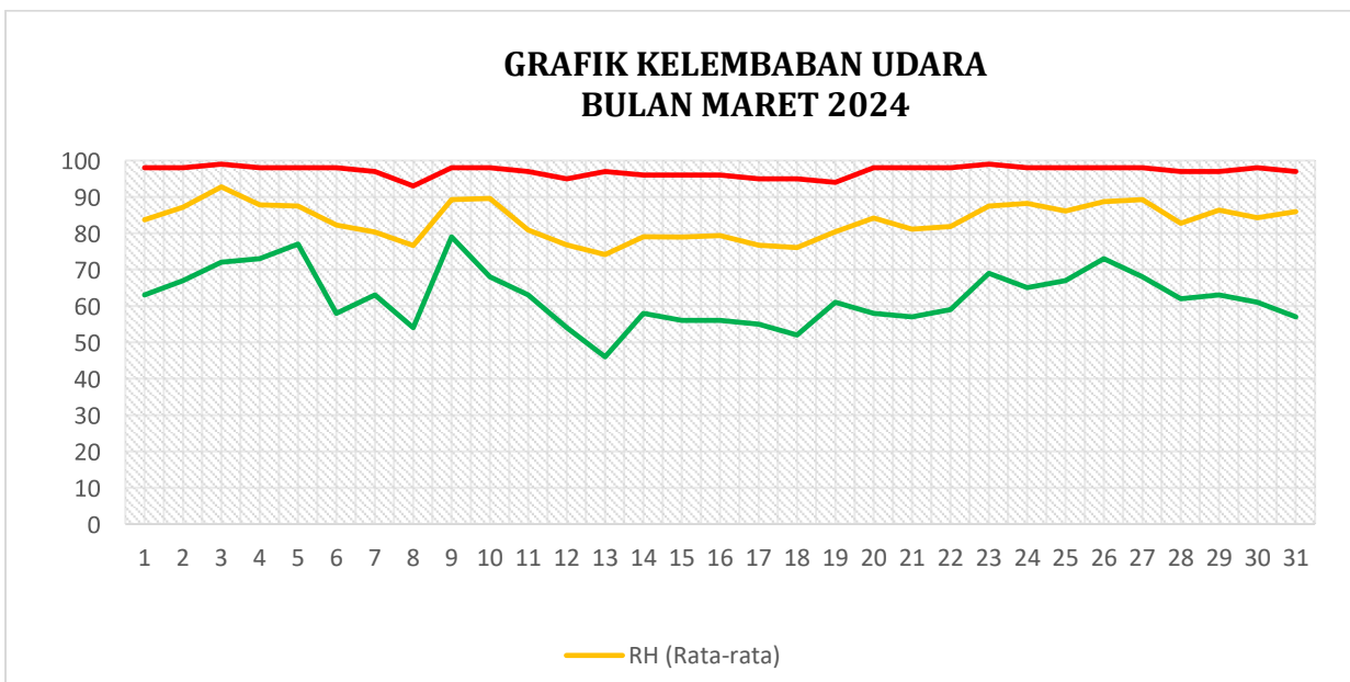
Gambar 2.1.5.1 Grafik Kelembaban Udara Bulan Maret 2024
