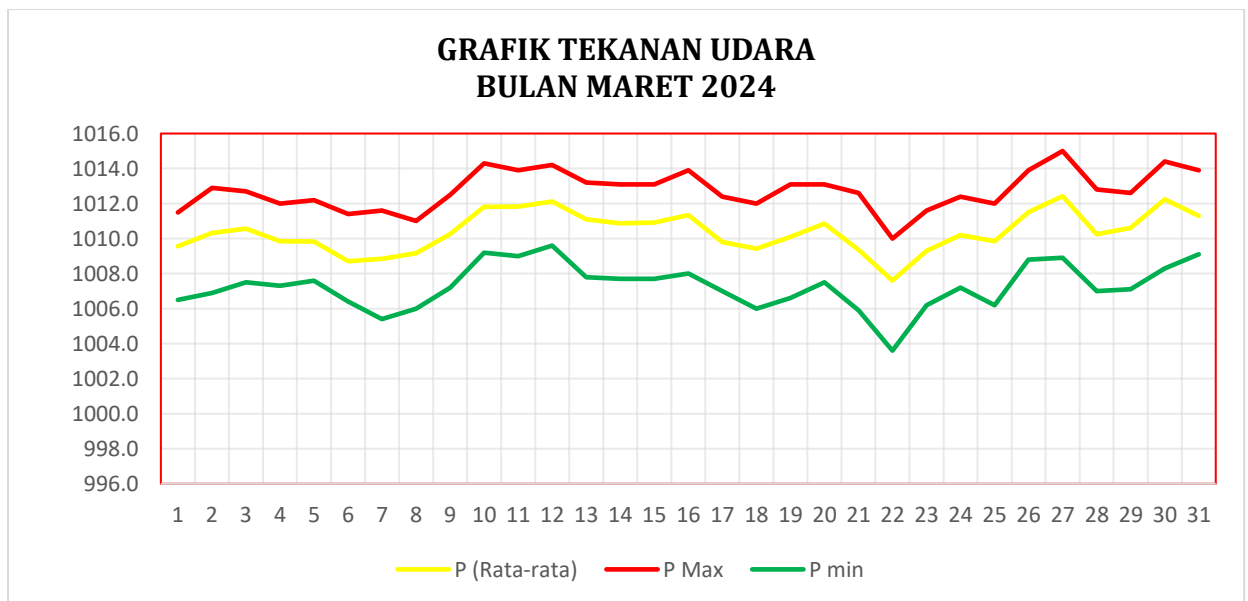
Gambar 2.1.4.1 Grafik Tekanan Udara Bulan Maret 2024
