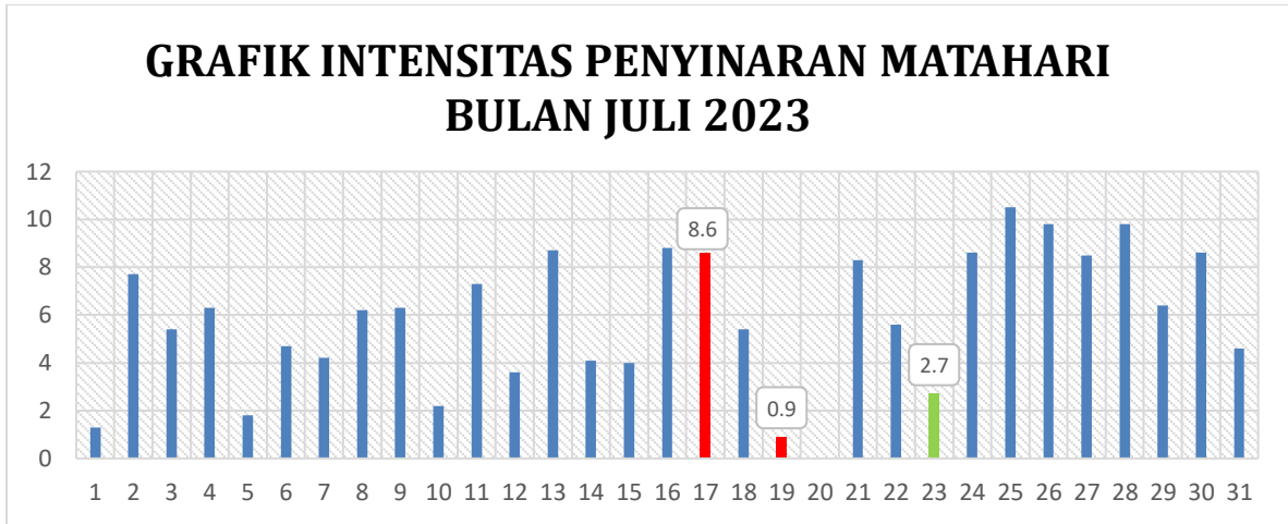
Gambar 2.1.2.1 Grafik Durasi Penyinaran Matahari Bulan Juli 2023
