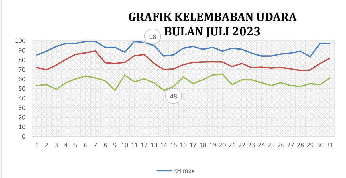
Gambar 2.1.5.1 Grafik Kelembaban Udara Bulan Juli 2023
