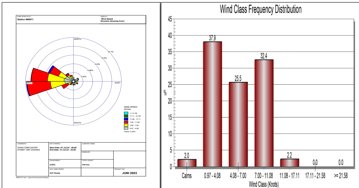
Gambar 2.1.6.1 Diagram dan Windrose bulan Juli 2023
