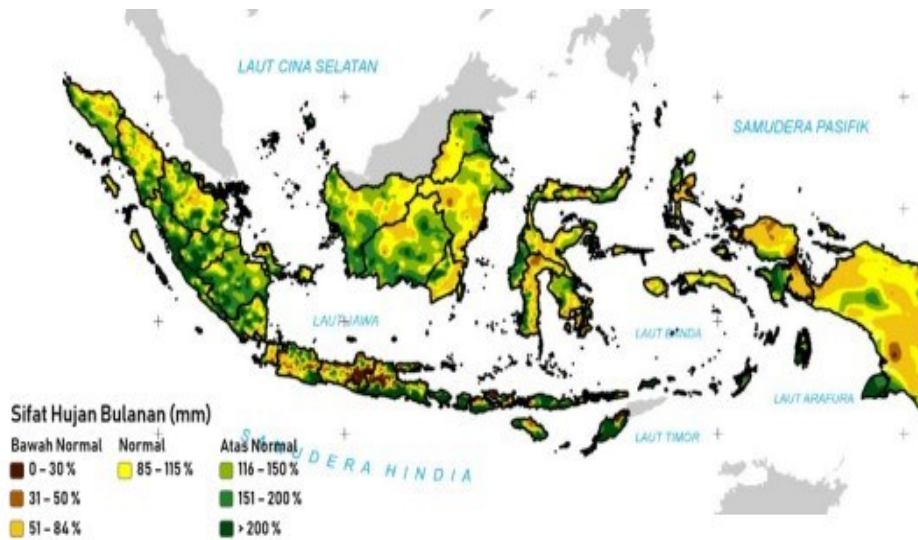
Gambar 1.2.5 Peta Analisis Sifat Hujan Bulan Juli 2023
