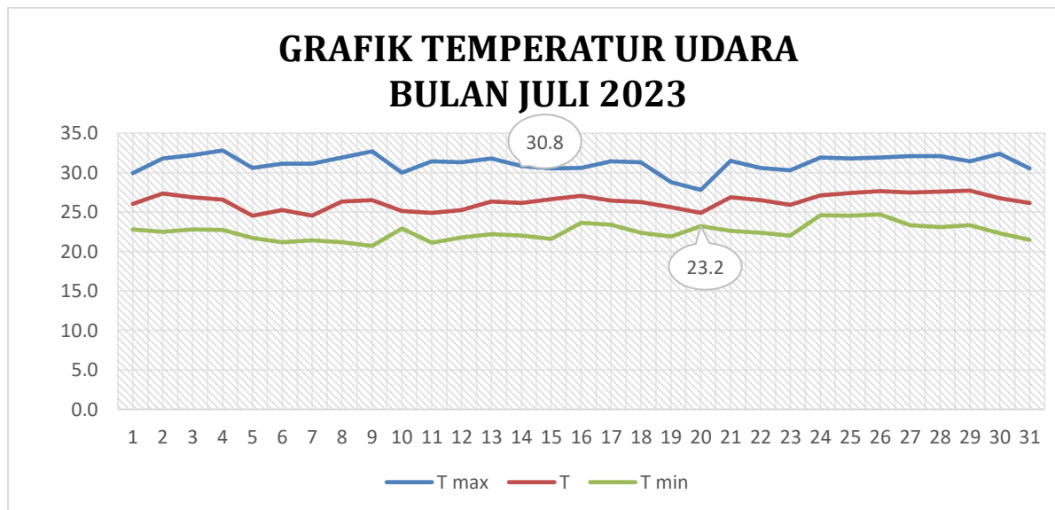
Gambar 2.1.1.1 Grafik Suhu Udara Bulan Juli 2023
