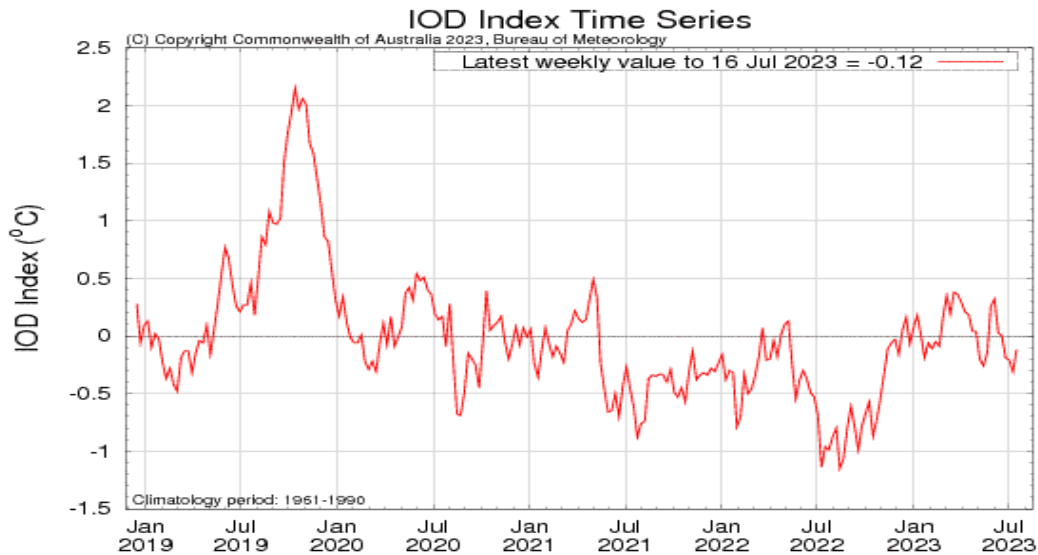
Gambar. 1.2.2 Indeks IOD Bulan Juli 2023
