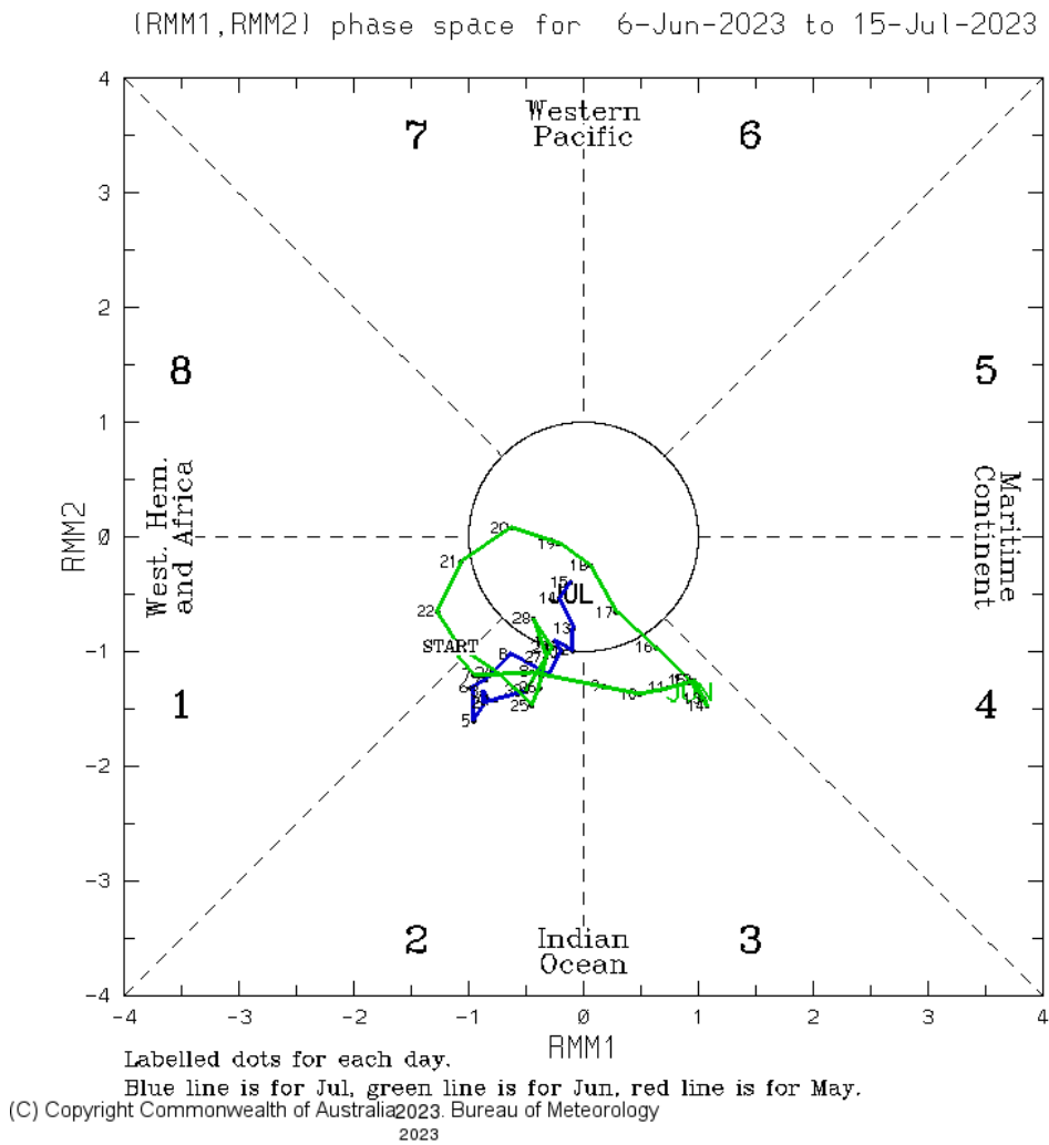
Gambar 1.2.6 Peta MJO Bulan Juli 2023
