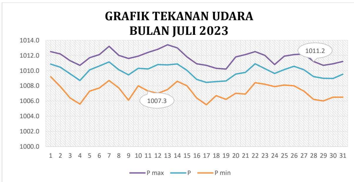
Gambar 2.1.4.1 Grafik Tekanan Udara Bulan Juli 2023
